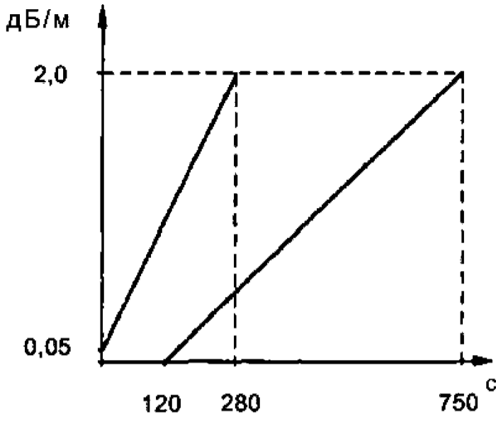
Рисунок Л.3 – Предельные значения зависимости m от t
