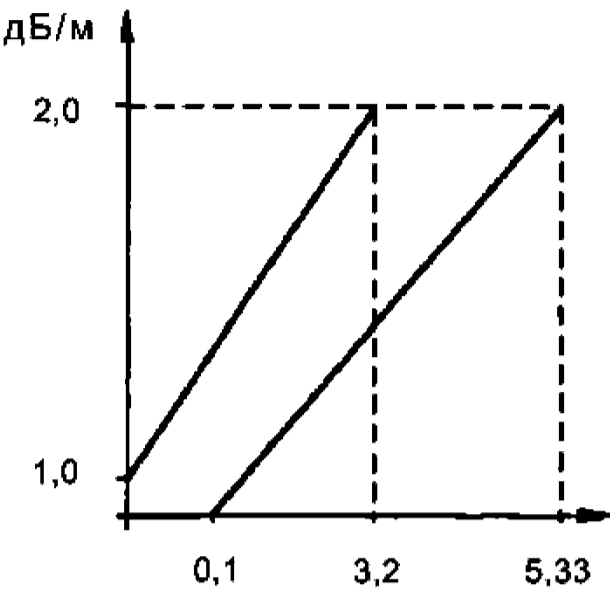
Рисунок Л.2 – Предельные значения зависимости m от y
