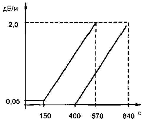
Рисунок К.3 – Предельные значения зависимости m от t
