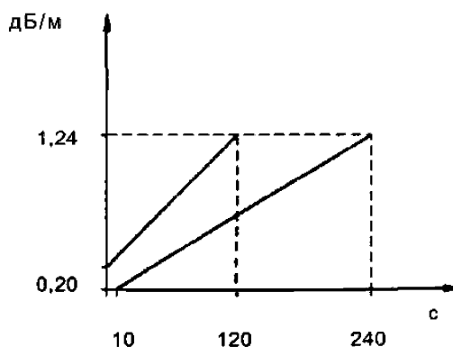
Рисунок Н.3 – Предельные значения зависимости m от t
