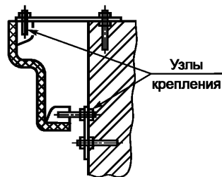
Рисунок 2 — Узел крепления СФБ изделия при вертикальной облицовке
