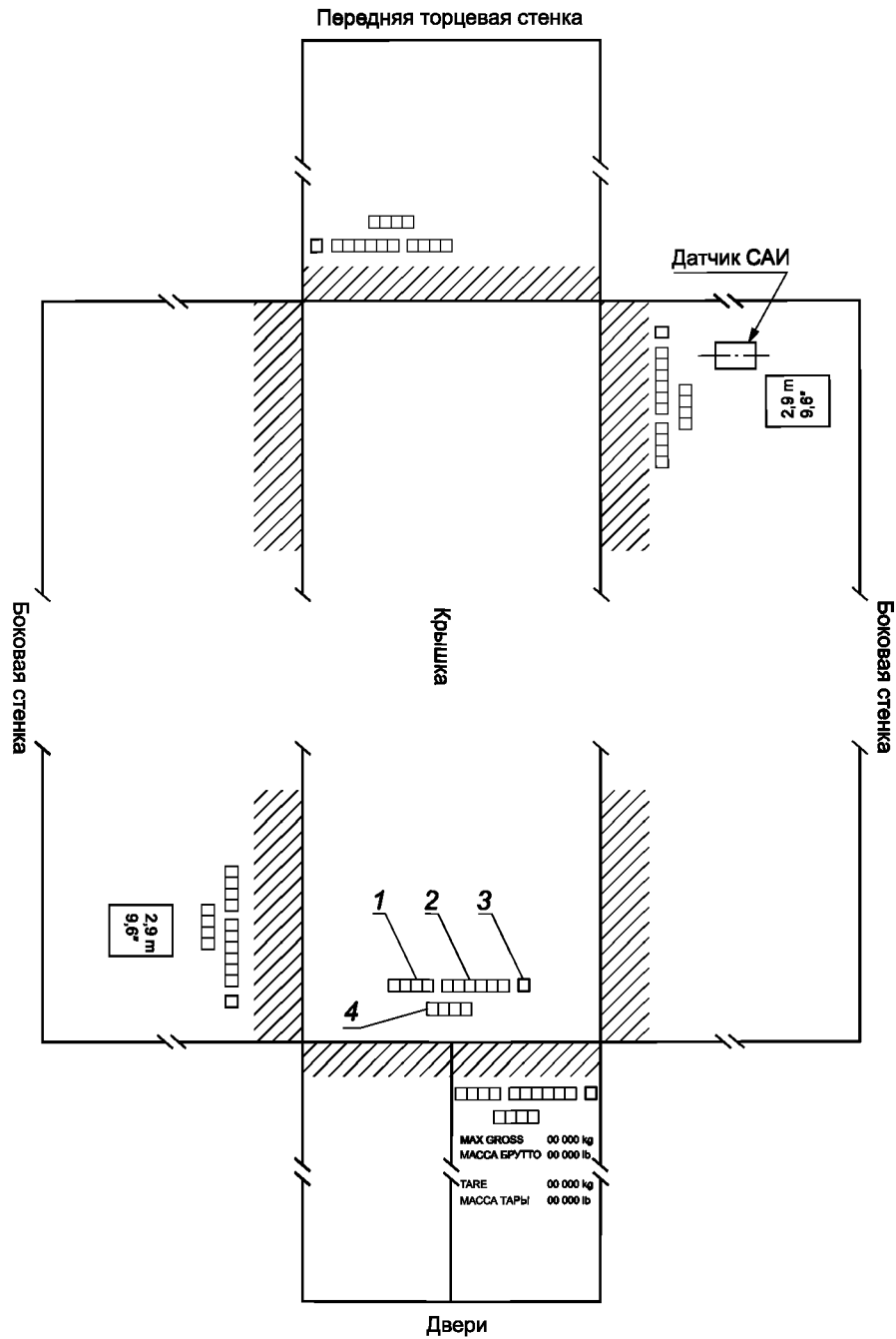
Рисунок Б.1 — Схема нанесения маркировки на внешнюю поверхность мобильного (инвентарного) здания
