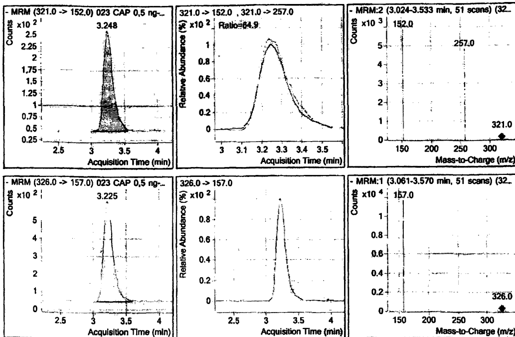
Рисунок 1 - Хроматограмма и масс-спектр стандартного раствора левомицетина концентрацией 0,5 \text{ нг/см}^3 содержащего внутренний стандарт левомицетин-d5 концентрацией 1 \text{ нг/см}^3
