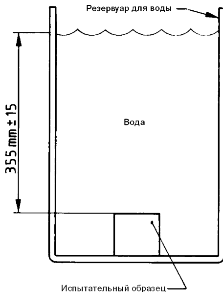
Рисунок 1 — Резервуар для воды при проведении испытаний герметичности приборов
