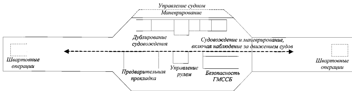
Рис. 2.5.17-3 Принципы проектирования — плоская фронтальная стенка — открытые крылья мостика с проходом от двери к двери.
