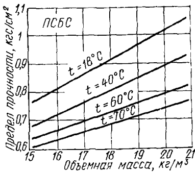
РИС. 43. ЗАВИСИМОСТЬ ПРЕДЕЛА ПРОЧНОСТИ ПРИ СЖАТИИ ОТ ОБЪЕМНОЙ МАССЫ БЕСПРЕССОВЫХ ПОЛИСТИРОЛЬНЫХ ПЕНОПЛАСТОВ ПРИ РАЗЛИЧНЫХ ТЕМПЕРАТУРАХ
