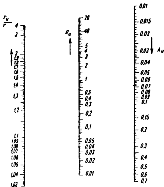
Рис. 3. Номограмма для определения термического сопротивления кольцевой теплоизоляции трубопровода R_{ж}
