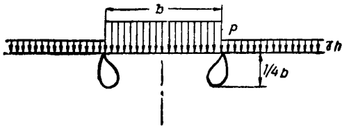
Рис. 19. Схема областей местного нарушения прочности основания
