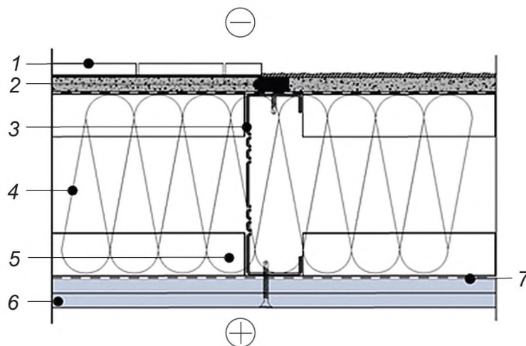
1 — облицовка (фасадная отделка); 2 — самонарезающие винты для соединения обшивки с элементами каркаса; 3 — стойки каркаса стены; 4 — основной теплоизоляционный слой (между стойками каркаса); 5 — противоусадочные уголки; 6 — внутренняя обшивка КОС; 7 — пароизоляция
