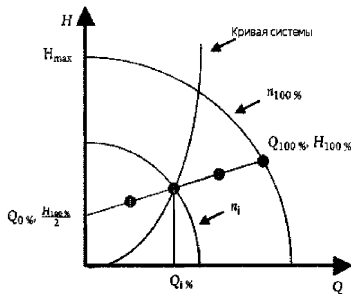
Рис. 2. Кривая системы интегрированного циркуляционного насоса.
