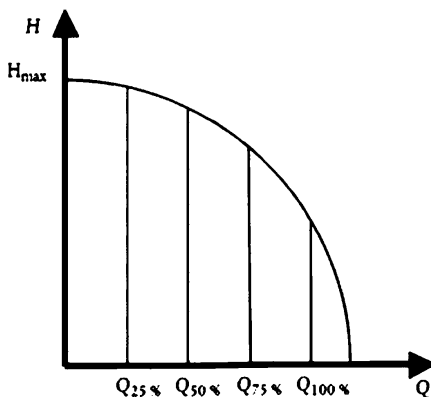
Рис. 3. Профиль нагрузки.
