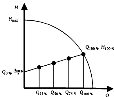
Рис. 1. Опорная контрольная линия циркуляционного насоса.
