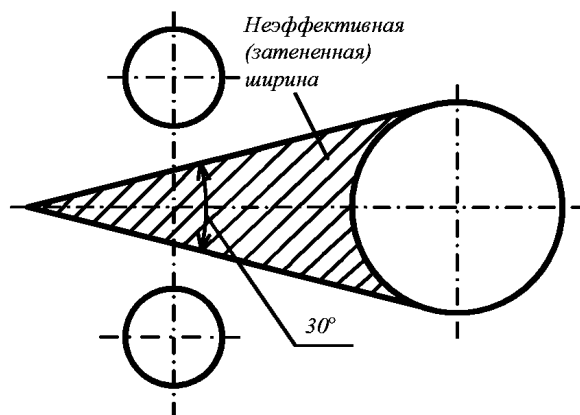
Рис. 1.4.8.3 Расчетное сечение
