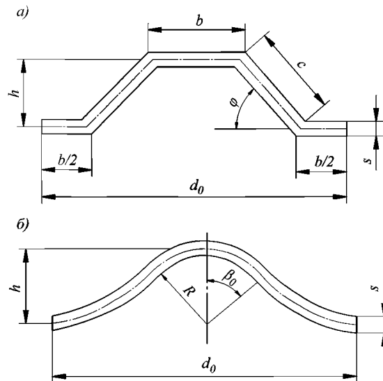
Рис. 1.6.4.5.1 Коробчатые ( a ) и волнистые ( б ) гофры
