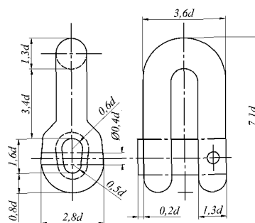
Рис. 7.1.3-5 Соединительная скоба
