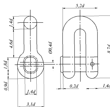
Рис. 7.1.3-6 Концевая скоба
