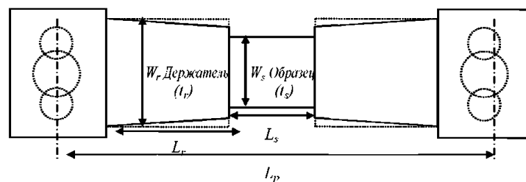
Рис. 3.20.6.2 Схема расположения испытываемого образца, держателя и оснастки
