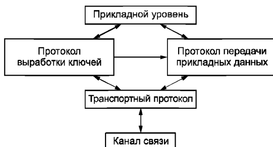
Рисунок 1 — Схема информационного обмена
