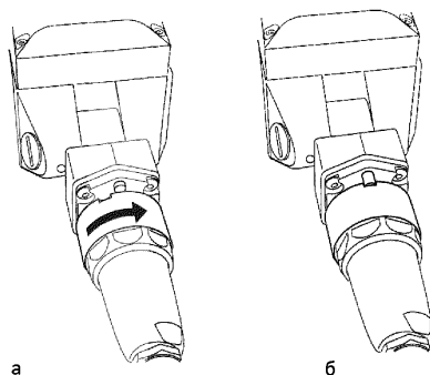
а – направление заворачивания разъема, б – закрепление фиксатора в пазу
