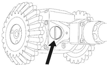
Рисунок А.5 – Клапан заправки азота на транспортном модуле
