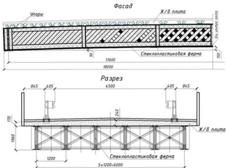
Рисунок В.3 – Схематический чертеж автодорожного пролетного строения
