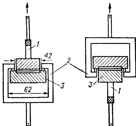
Приспособление для закрепления образцов при испытании на равномерный отрыв:
