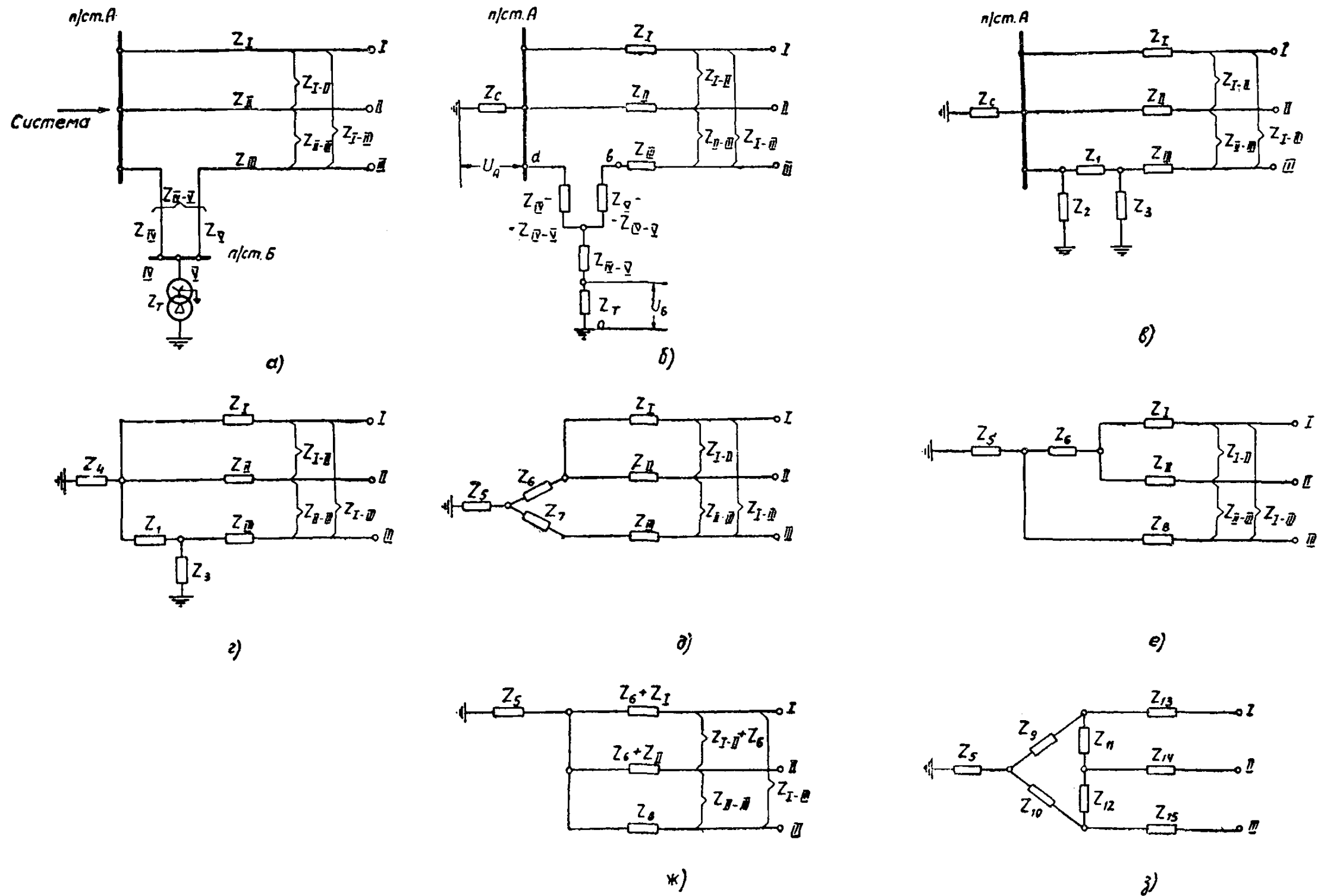
Рис. П-18. Схема замещения нулевой последовательности трех параллельных линий с одной общей точкой и петлевым отвлечением от одной из них. Примечания: 1. Z_c — суммарное сопротивление нулевой последовательности системы. 2. U_A, U_B — напряжение нулевой последовательности на шинах n/cт. A и n/cт. B .
