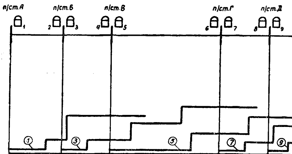
Рис. 6. Пример согласования характеристик токовых защит.
