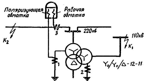
а) Схема включения реле
