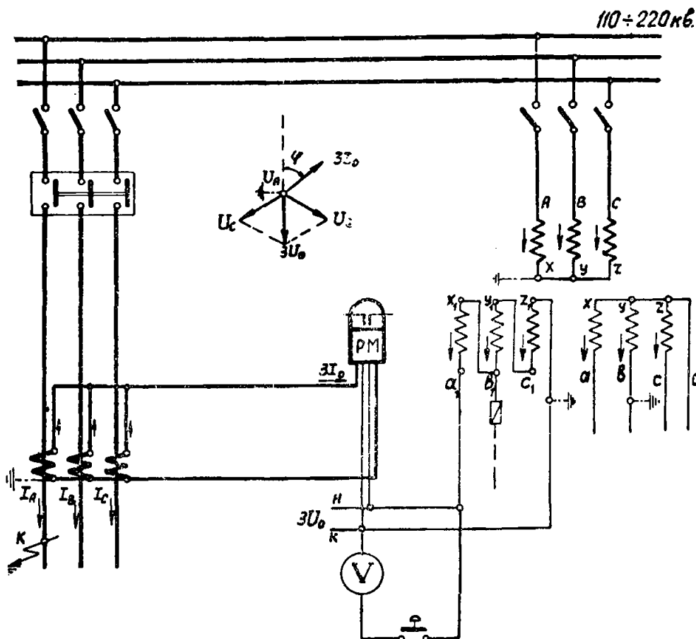
Рис. 5. Принципиальная схема присоединения реле направления мощности нулевой последовательности к трансформаторам тока и напряжения и схема периодического контроля цепей напряжения.
