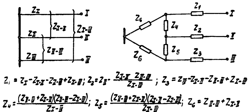
Рис. П-9. Схемы замещения нулевой последовательности двух и трех параллельных линий, имеющих общую точку с одного конца.
