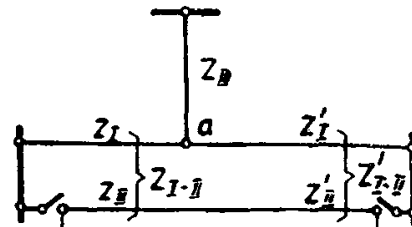
б) Исходная схема и схема замещения двух параллельных линий, одна из которых имеет заход шлейфом на подстанцию, а другая заземлена с обоих концов.
