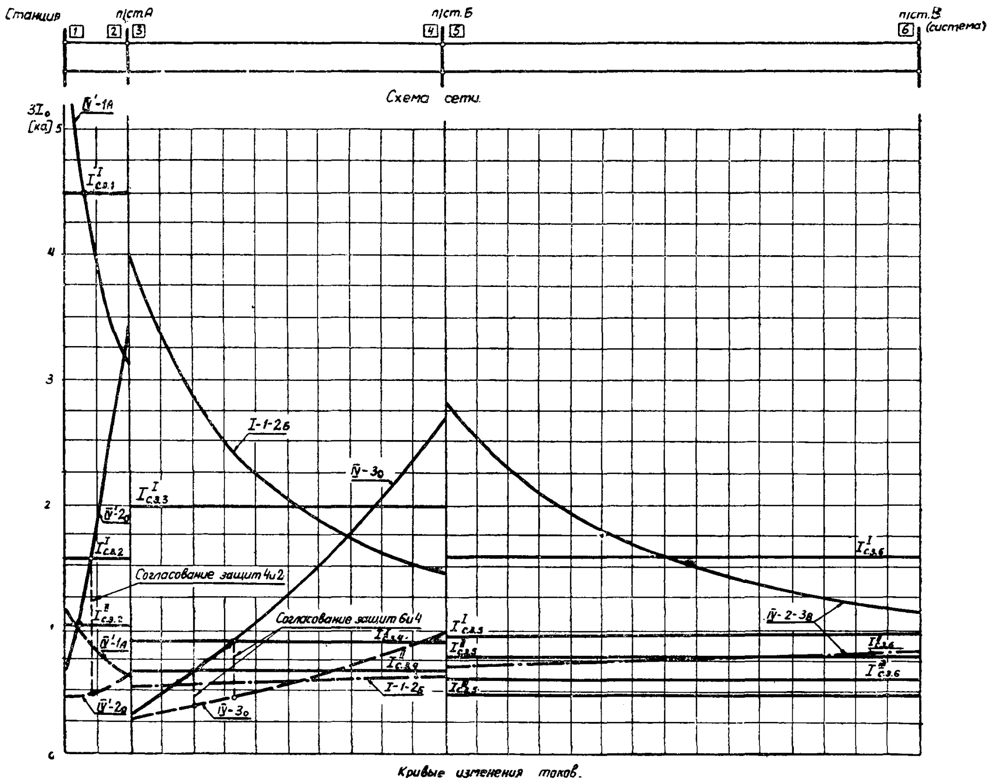
Рис. 21. Расчет токов срабатывания вторых ступеней защит 2, 4, 6 и третьей ступени защиты 6 в сети рис. 19.
