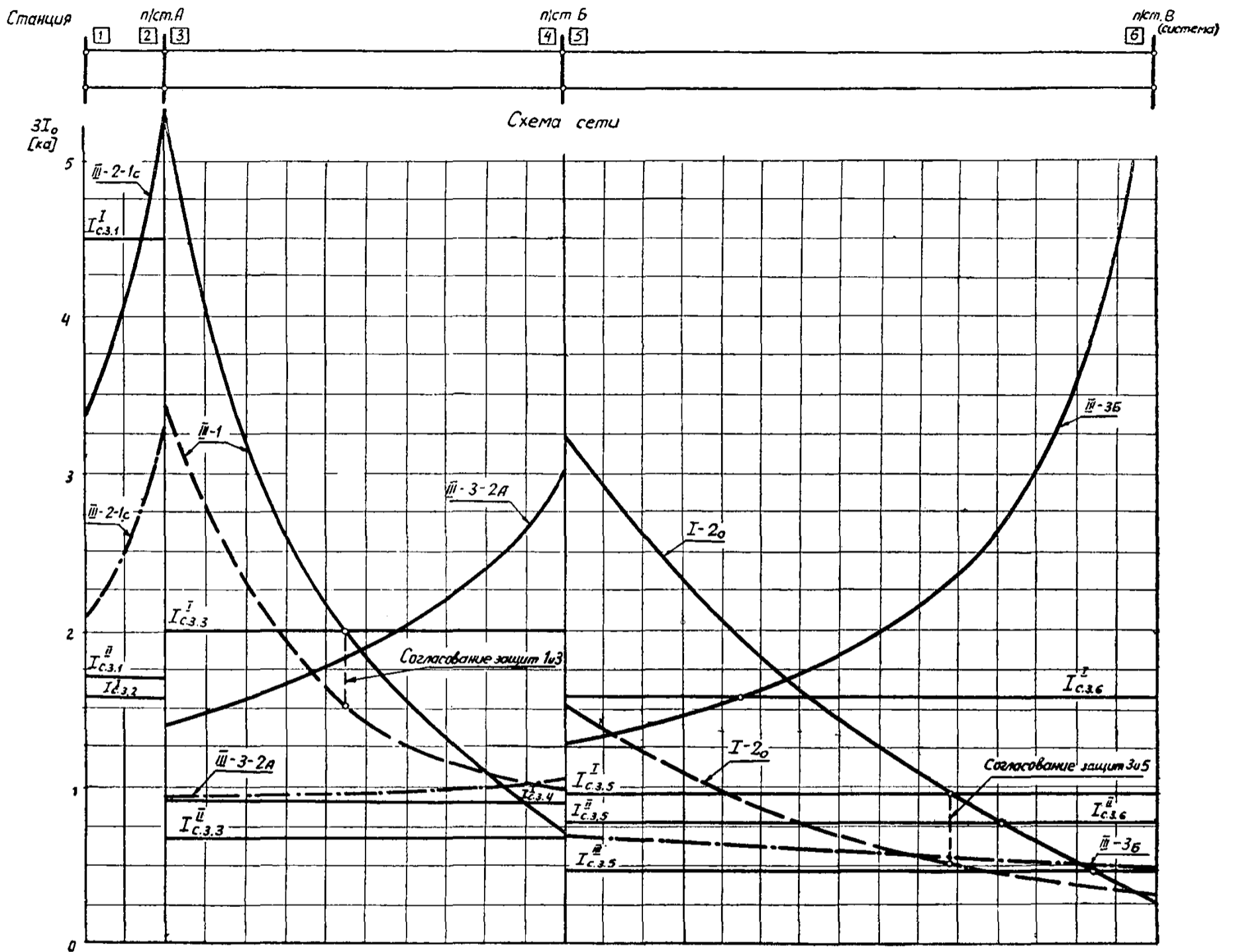
Кривые изменения токов.
