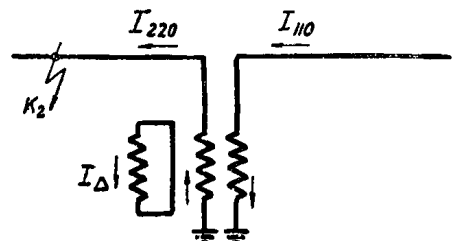
в) Замыкание в точке K_2 (схемы «а»)
