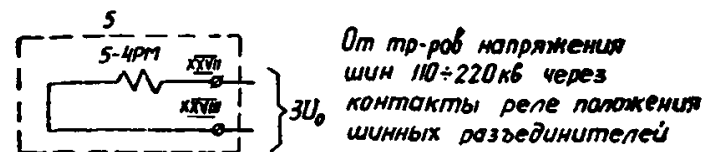
в) Цели напряжения
