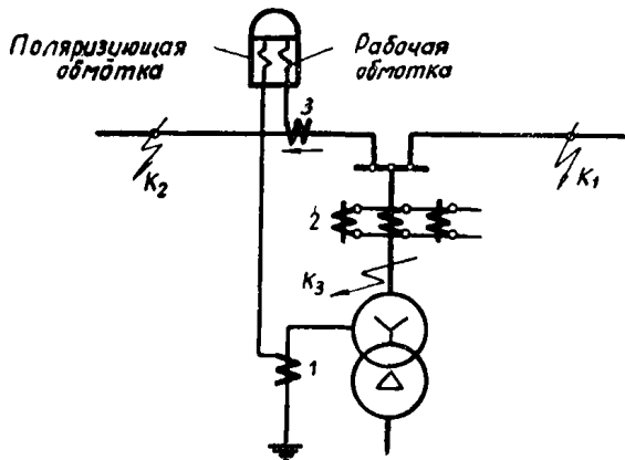
Рис. П-1. Включение поляризирующей обмотки реле направления мощности на ток в нейтрали двухобмоточного трансформатора.
