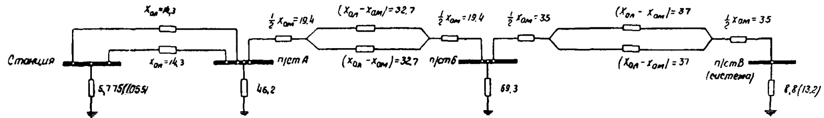
в) Схема замещения нулевой последовательности
