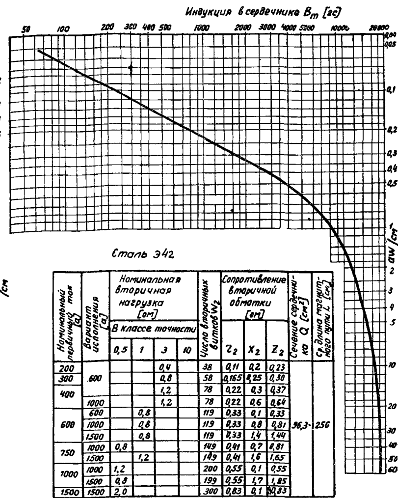
Трансформаторы тока типа ТВД220 (Данные завода "Уралэлектроаппарат").
