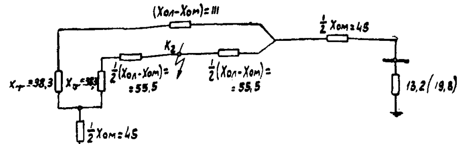
в-2) Схема замещения нулевой последовательности при к.з. на землю в точке K_2
