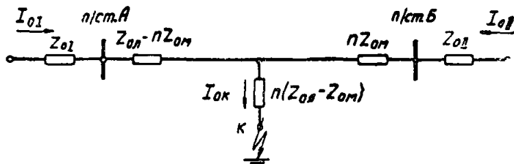
б) Схема замещения нулевой последовательности.
