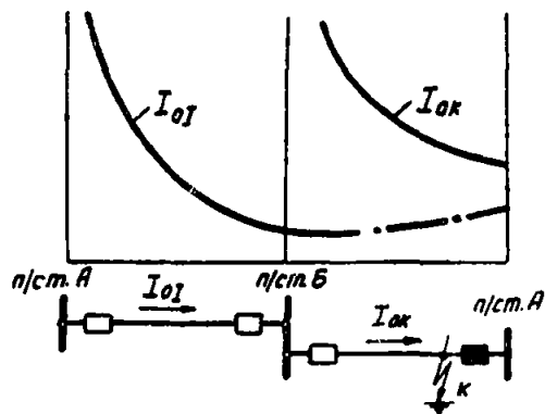
в) Пример изменения токов в поврежденной и неповрежденной линиях.
