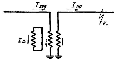
б) Замыкание в точке K_1 (схемы «а»)
