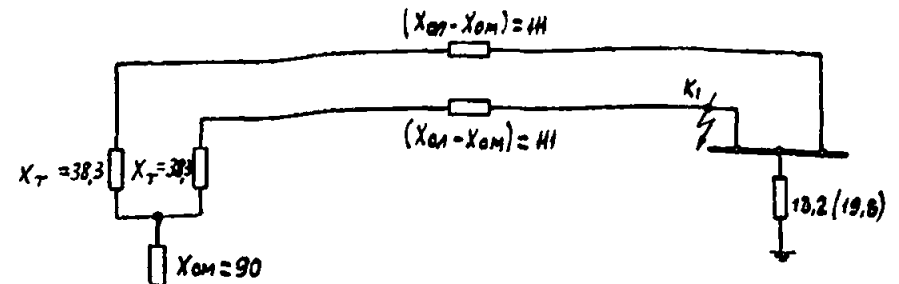
в-1) Схема замещения нулевой последовательности при к.з. на землю в точке K_1
