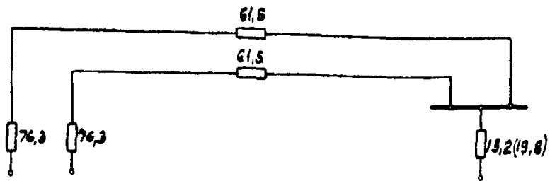
б) Схема замещения прямой (обратной) последовательности.
