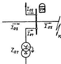
б) Пример определения Z_{0c} при заданном токораспределении.
