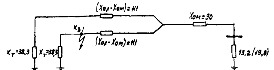
в-3) Схема замещения нулевой последовательности при к.з. на землю в точке K_3
