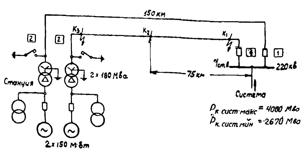
а) Исходная схема.
