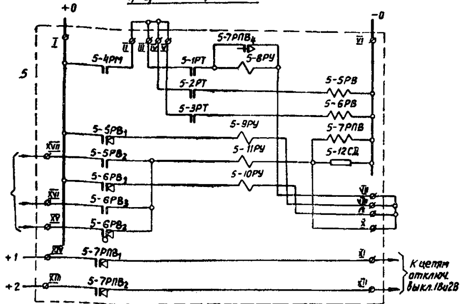
г) Цели оперативного постоянного тока
