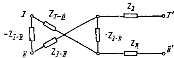
б) Схема замещения рис. „а“ (вариант 1)
