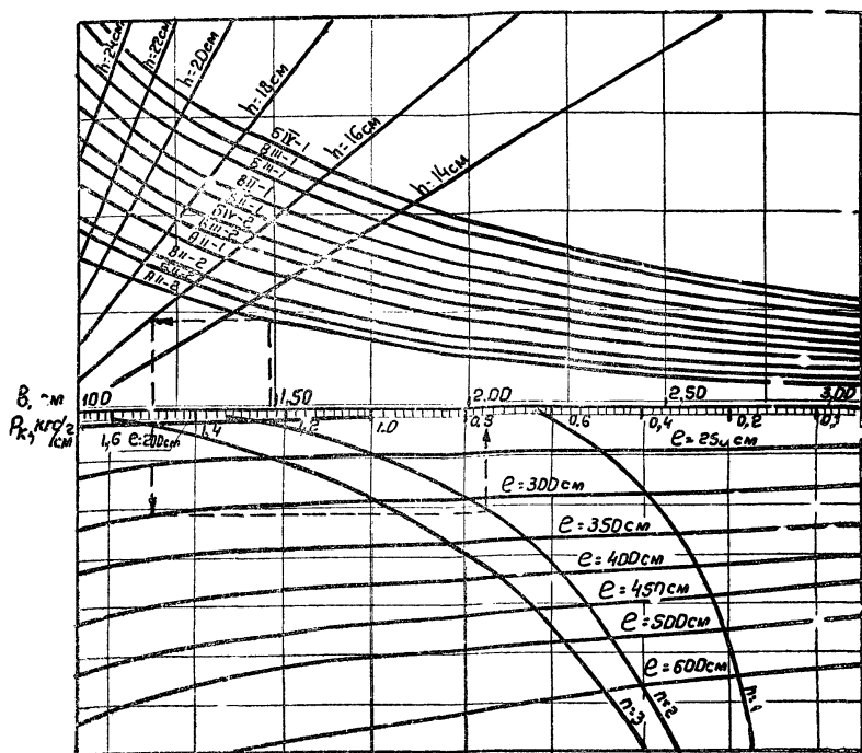
Рис. 53. Номограмма для определения величины максимального давления ( P_k ) на поверхность основания от колеса расчетного автомобиля с осевой нагрузкой 10 т
