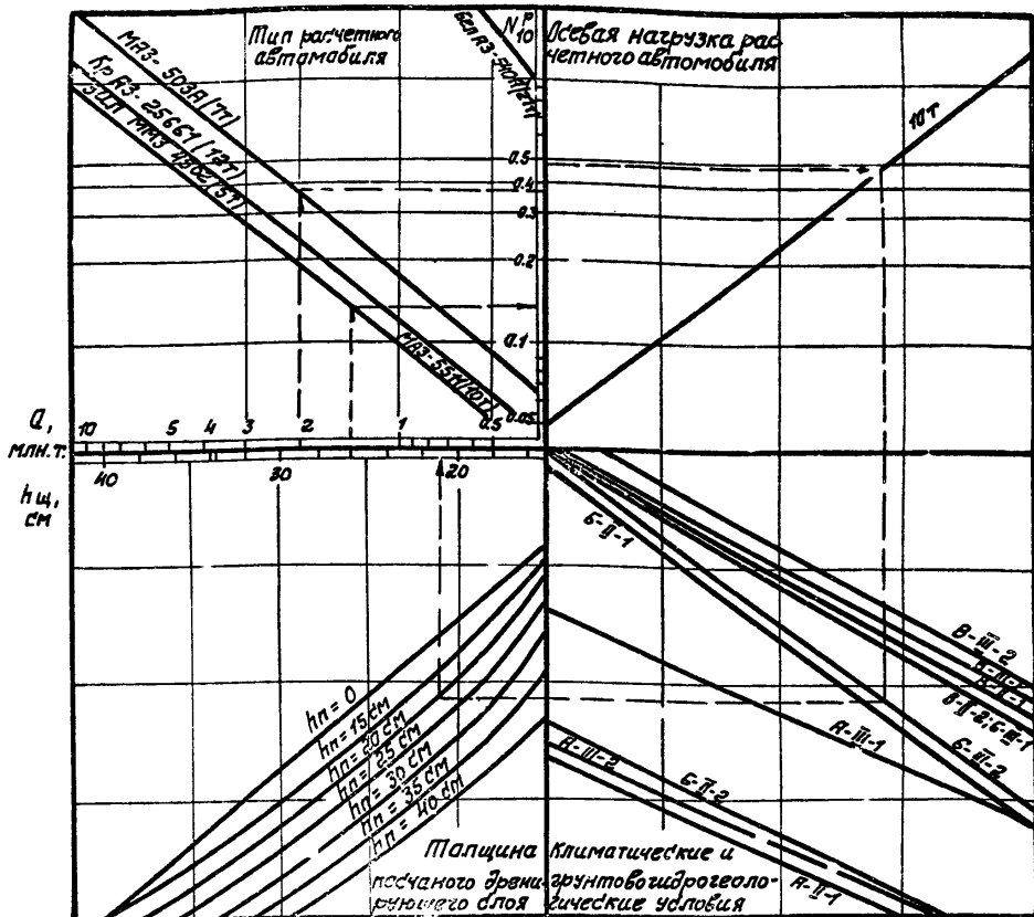
Рис. 5.9. Номограмма для определения толщины щебеночного основания канструкций дорожных одежд с покрытием из черного щебня при расчетном автомобиле с осевой нагрузкой 10 т
