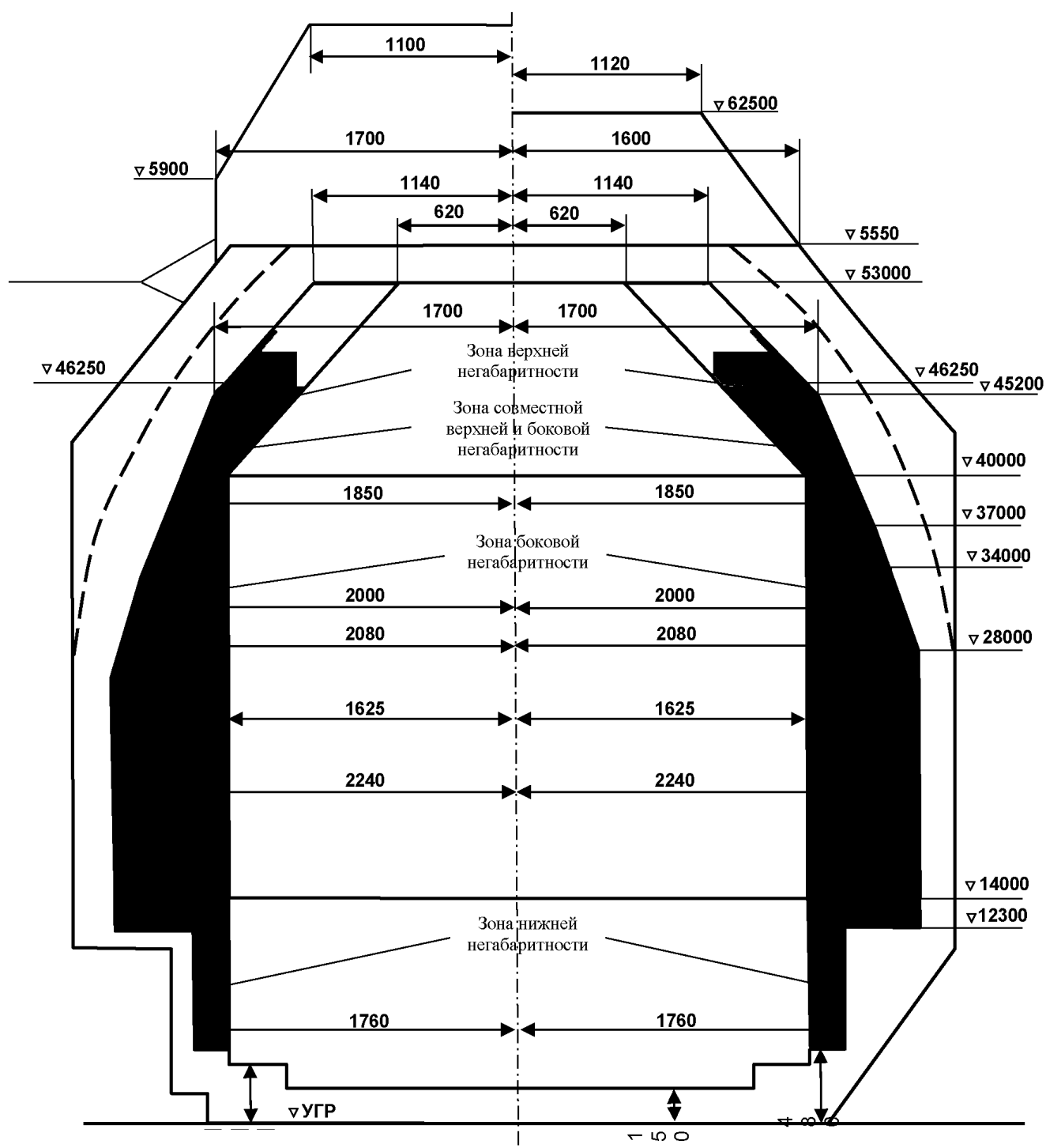
Рис.1. Зоны негабаритности груза
