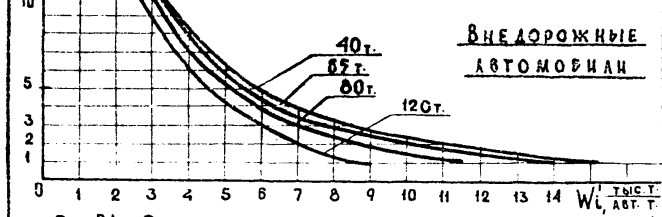
Рис.31 Средняя годовая производительность автомобилей
