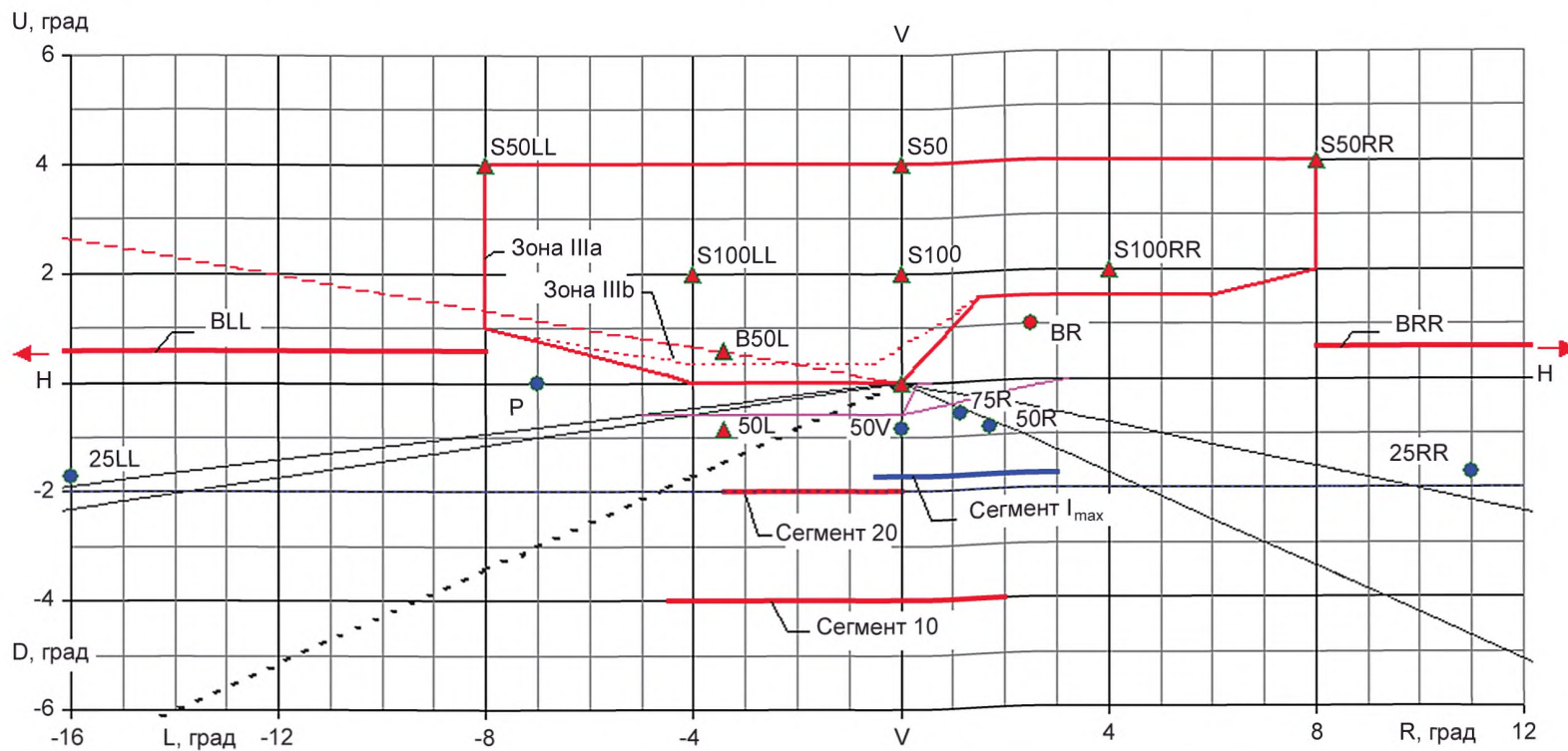
Рисунок Б.1— Фотометрические требования в отношении угловых положений луча ближнего света (для правостороннего движения)
