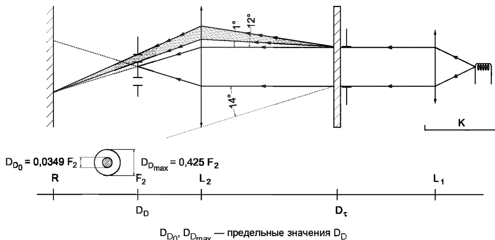
Рисунок В.1 — Оптическая система для измерения изменений рассеивания и пропускания света
