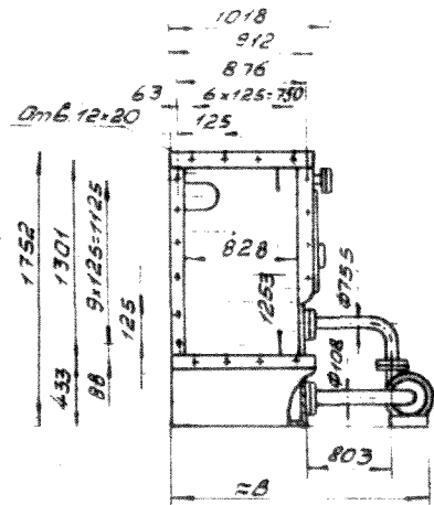
КТЦ 2-315; КТЦ 2-40; КТЦ 2-63; КТЦ 2-80.
