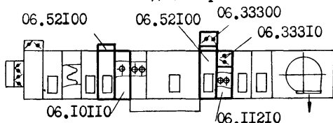
Схема кондиционера
