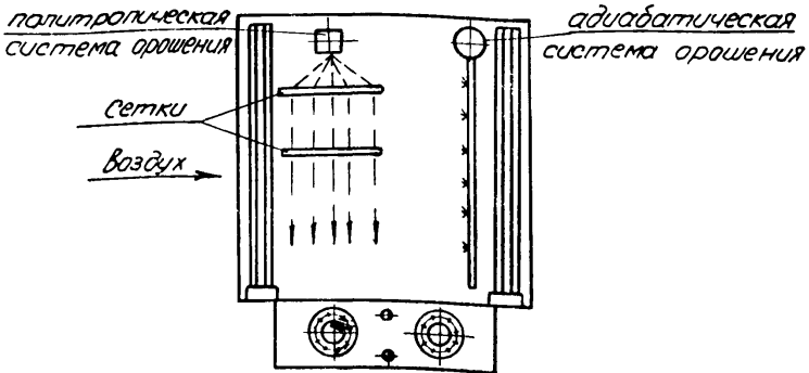
Схема камер орошения ОКС-2 КТЦ2-315; КТЦ2-40; КТЦ2-63; КТЦ2-80
