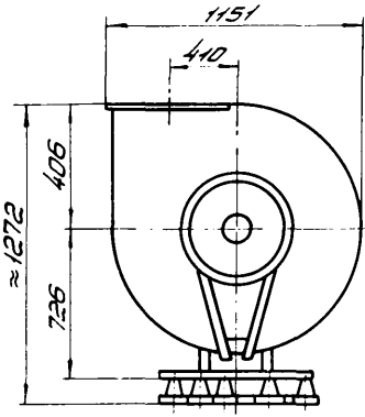
Вид А
