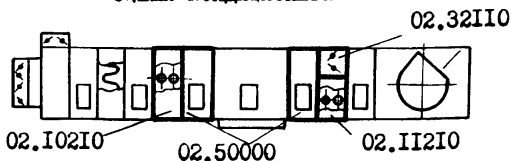
СХЕМА КОНДИЦИОНЕРА
