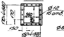
Вид Д
