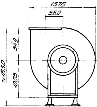
Вид Д
