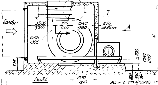
Рис. 1 воздух ↑ ось отв. выхлоп вверх
