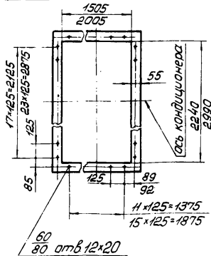
Вид Б; Вид Б, повернуто
