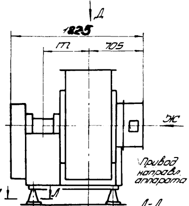
Л-Л
