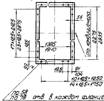
В-В Фланцы - нижний и верхний прямоугольного перехода
