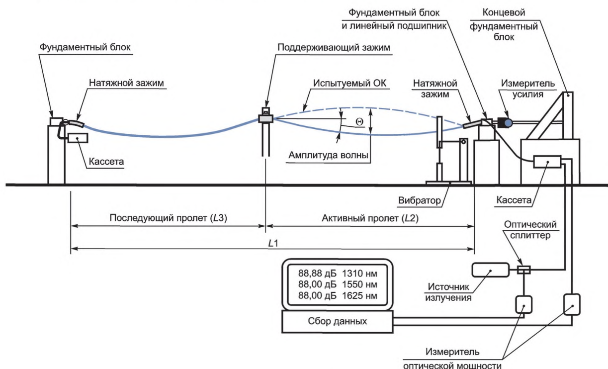
Рисунок 33 — Схема испытания ОК на галопирование (пляска ОК)
