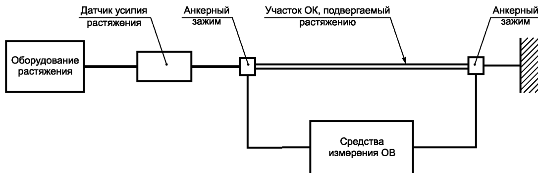
Рисунок 1 — Схема стенда для испытания ОК на растяжение
