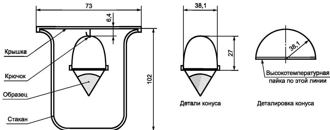
Рисунок 18 — Оснастка для испытания на стекаемость и испарение
