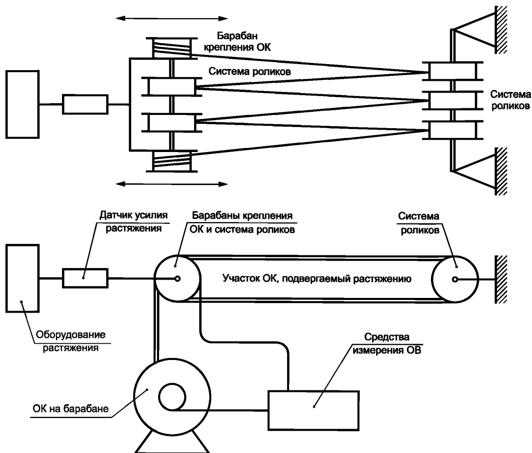
Рисунок 2 — Пример схемы стенда для испытания ОК на растяжение с использованием систем роликов и барабанов крепления ОК
