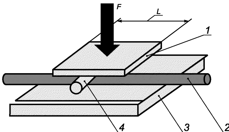
Рисунок 5 — Схема стенда для испытания на сдвливание, метод Е3А, детали плиты/исполнение плиты
