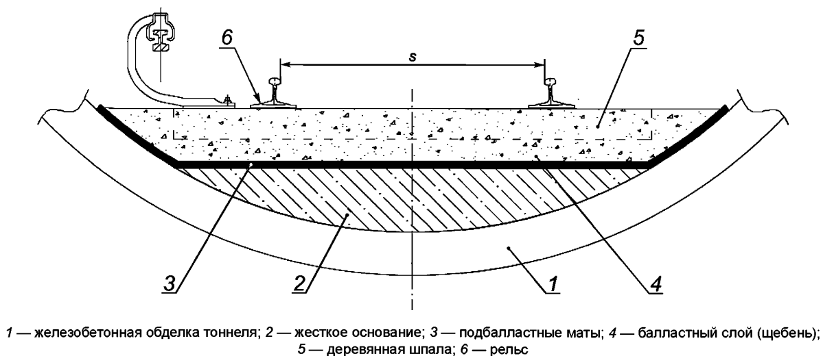
Рисунок В.7 — Поперечный профиль пути с подбалластными матами
