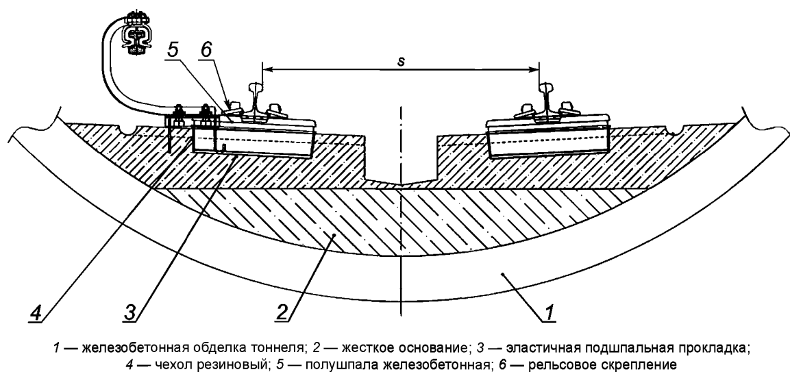
Рисунок В.6 — Поперечный профиль пути на железобетонных полушпалах с упругими подшпальными прокладками
