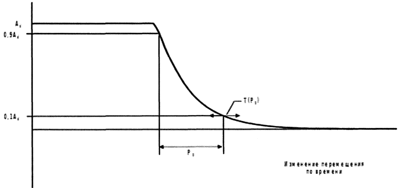
Схема 3. Характеристика переходного процесса с критическим демпфированием
