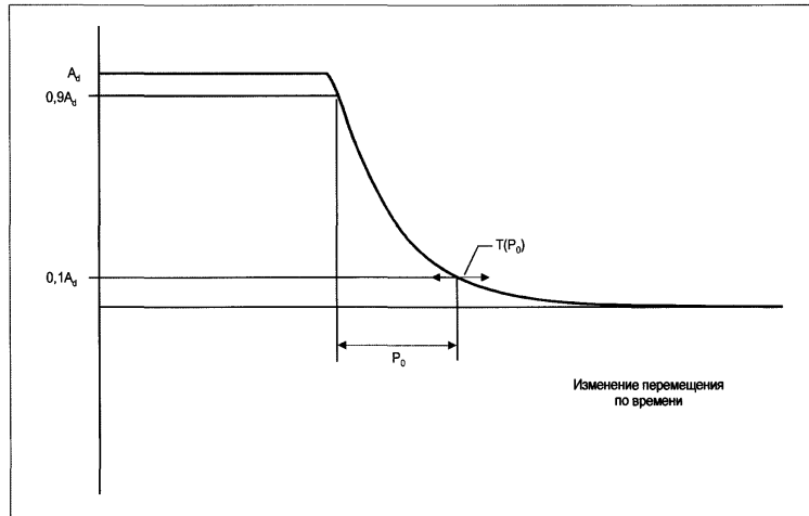
Схема 3. Характеристика переходного процесса с критическим демпфированием
