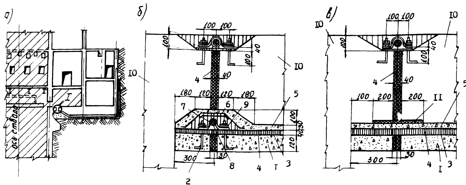
Рис. 6. Герметизация примыкания устья ствола к фундаментам копра: 1 — бетонная подготовка — 120 мм; 2 — анкерные болты; 3 — огрунтовка битумом; 4 — асфальт в два слоя с содержанием битума до 20%; 5 — цементный раствор состава 1:3; 6 — два слоя стеклоткани, пропитанной битумом; 7 — компенсатор из нержавеющей стали; 8 — просмоленный жгут; 9 — прижимная планка; 10 — железобетонная конструкция; 11 — прокладка из конвейерной ленты.
