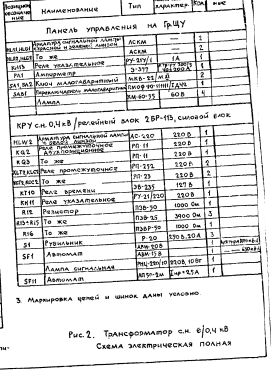
Рис. 2. Трансформатор с.к. 6/0,4 кВ Схема электрическая полная
