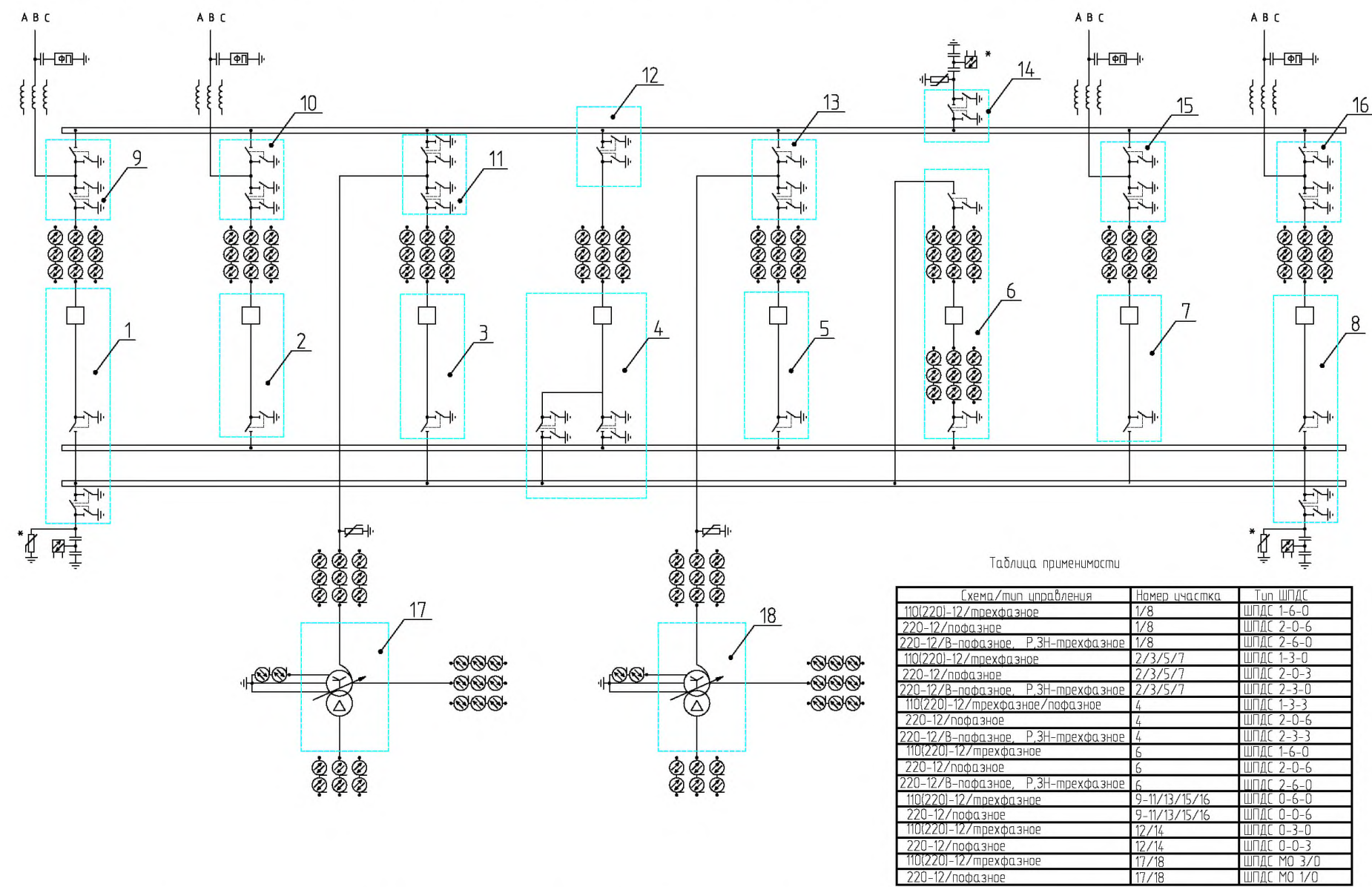
А.18 Схема № 12 – Одна рабочая, секционированная выключателем, и обходная системы шин
