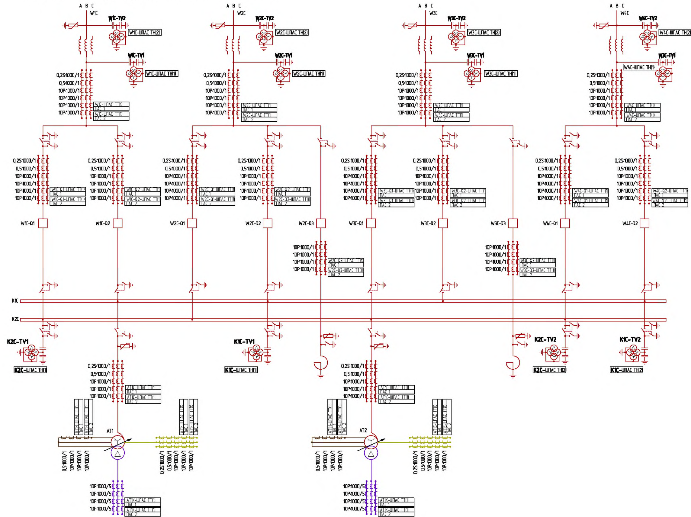
Схема Б.3 – Две рабочие системы шин
