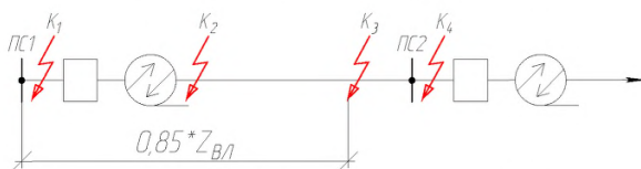
Рисунок 8.1. Схема для расчёта КЗ на присоединении ВЛ
