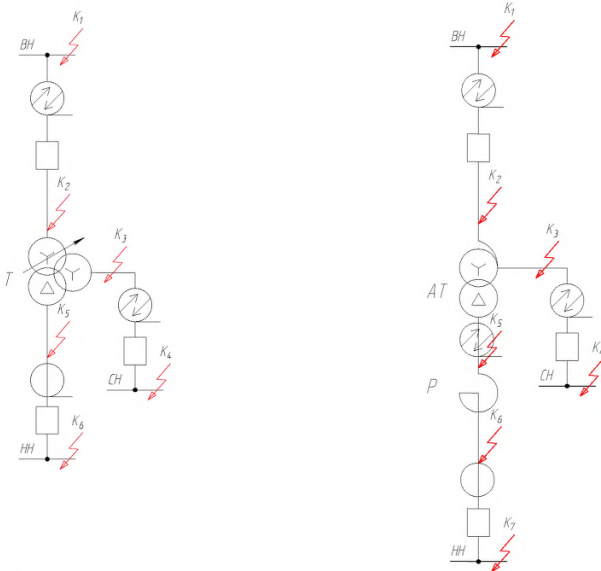
а) б) Рисунок 8.2. Схема расчёта токов КЗ на присоединении трансформатора (а) и автотрансформатора (б)
