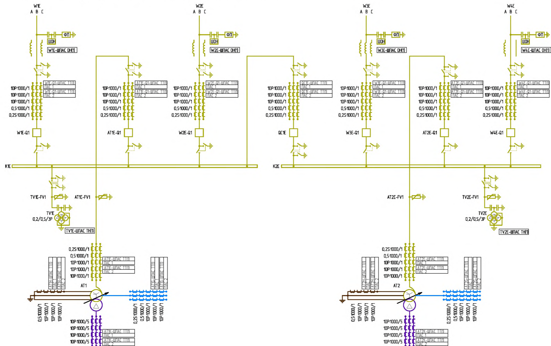
Схема Б.2 - Одна рабочая секционированная система шин
