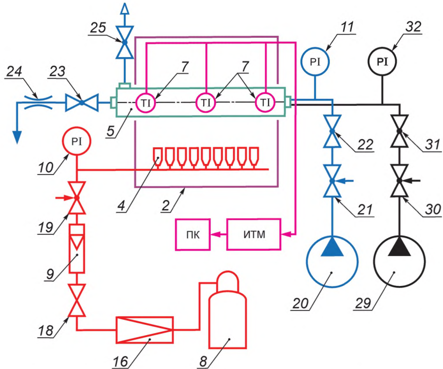
2 — испытательная камера; 4 — газовые горелки; 5 — трубопроводная сборка; 7 — термопары (ТІ); 8 — газовый баллон; 9 — расходомер; 10, 11, 32 — манометры (PI); 16 — редуктор; 18, 22, 23, 25, 31 — краны; 19, 21, 30 — регулирующие устройства; 20 — источник гидравлического давления; 24 — диафрагма; 29 — источник пневматического давления; ПК — персональный компьютер; ИТМ — многоканальный технологический измеритель
