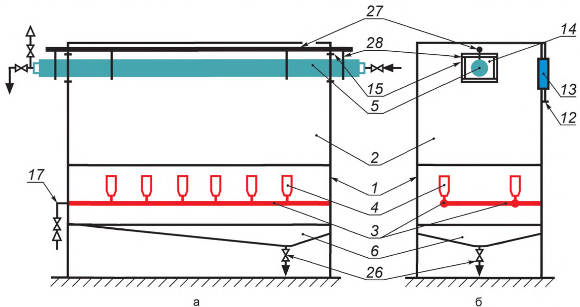
а — Фронтальный вид без передней стенки
