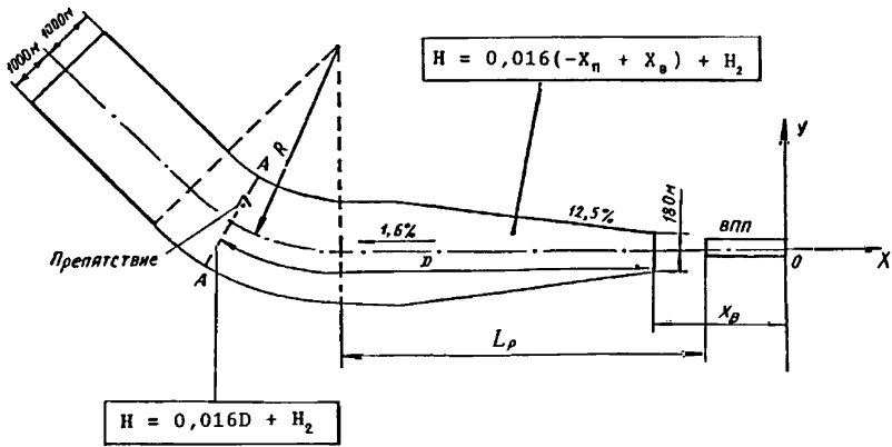
Рис. № 18. План поверхности взлета с отверстием (ВПП классов А, Б, В, Г).
