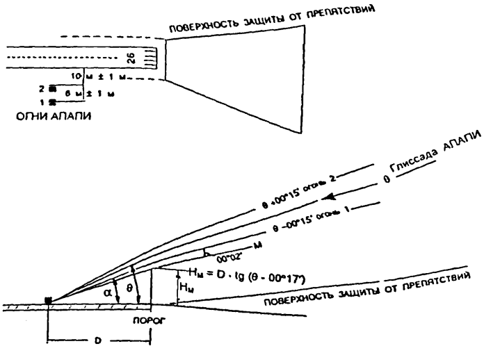
Рис. № 2. Размещение и углы возвышения световых пучков огней АРАРІ
