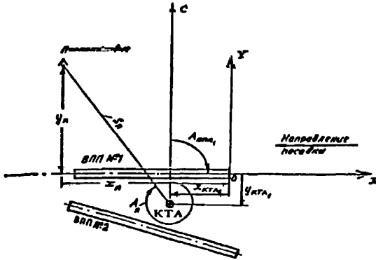
Рис. 2. Взаимное расположение полярной и прямоугольной системы координат
