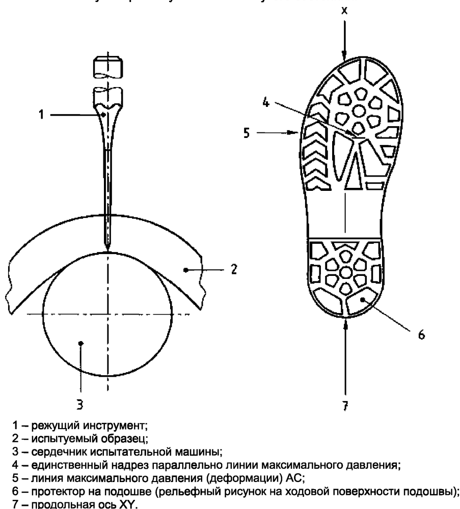
Рисунок 5 – Разрез подошвы
