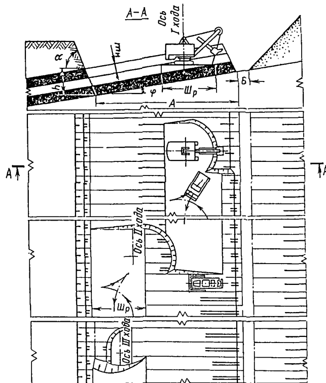
Схема 70 Технология разработки сближенных пластов поперечными ходами
