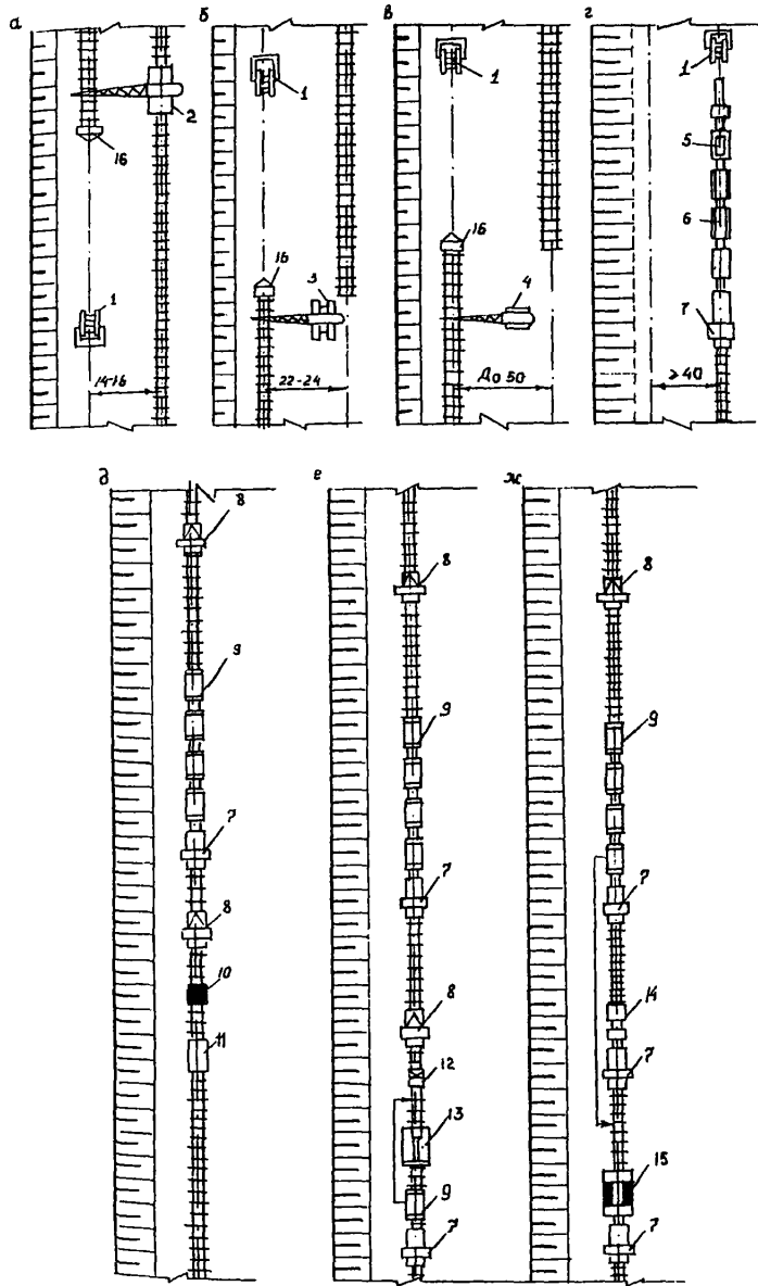
Рис. 18. Схемы путепереукладочных работ
