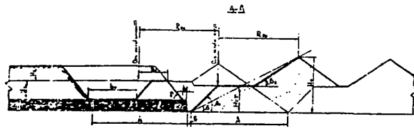
Технология разработки уступов драглайном широкими заходками
