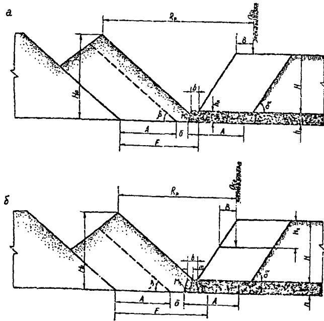
Рис. 5. Расчётные схемы для определения высоты первичного отвала и мощности обрабатываемой вскрыши при усложнённой бестранспортной системе:
