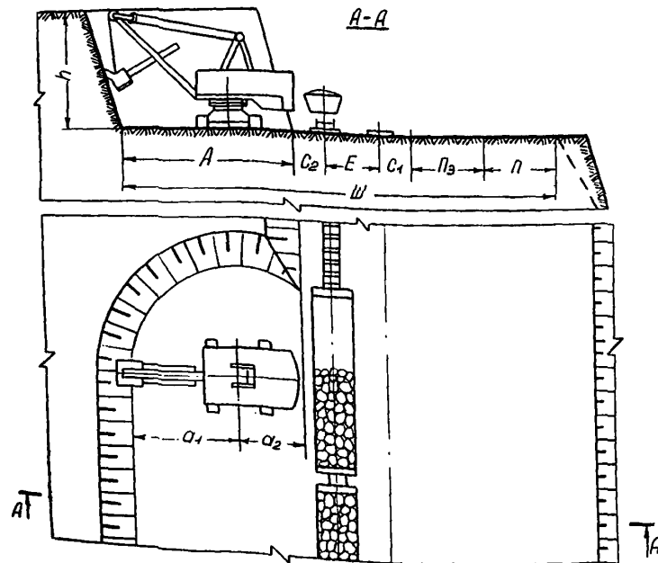
Схема I Технология разработки уступа
