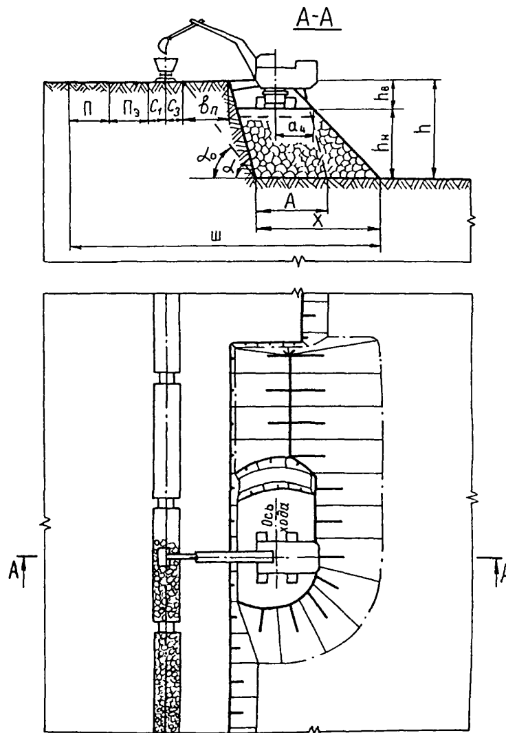
Технология разработки уступа обратной лопатой в два подступа
