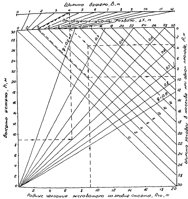
Рис.3. Номограмма для расчета параметров заходки
