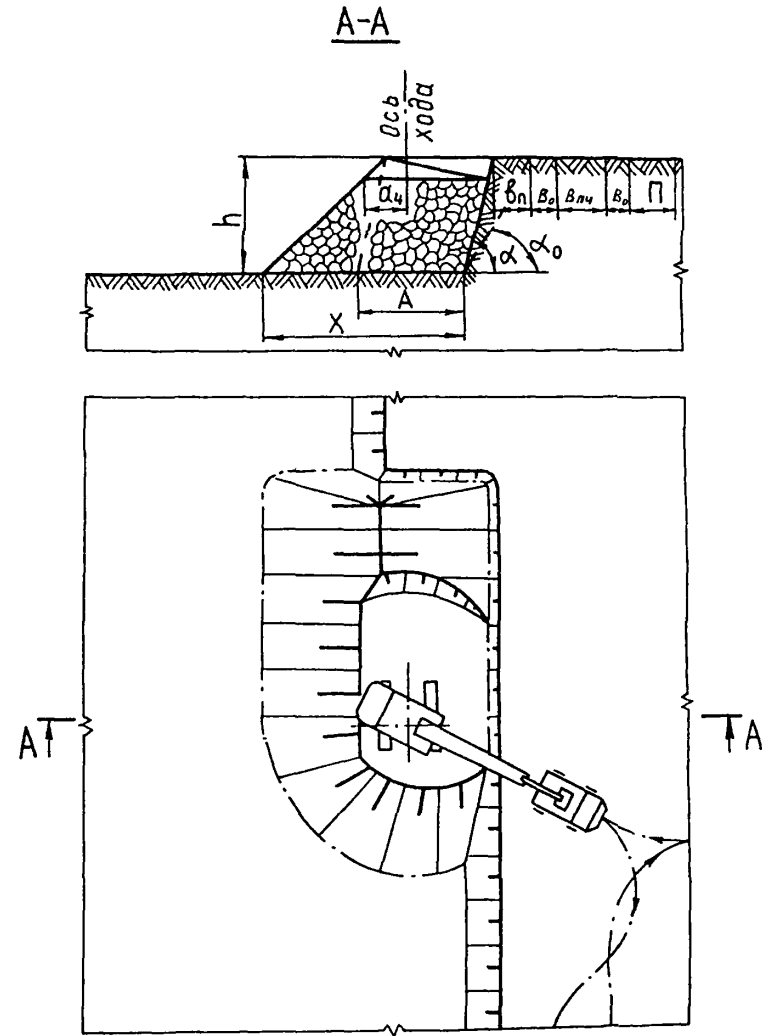
Технология разработки уступа обратной лопатой
