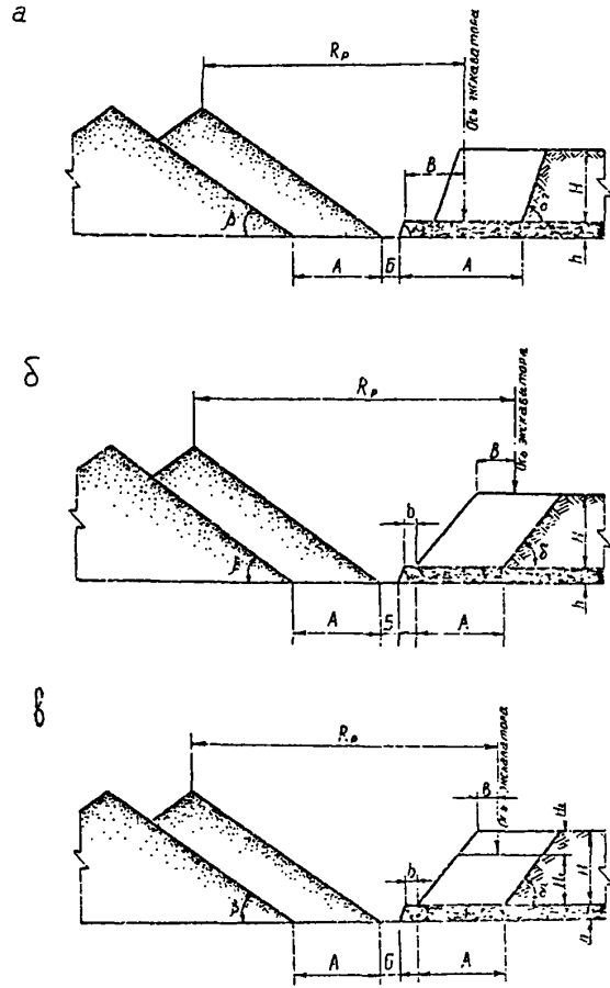
Рис. 2. Расчётные схемы для определения мощности вскрыши, обрабатываемой по простой бестранспортной системе разработки
