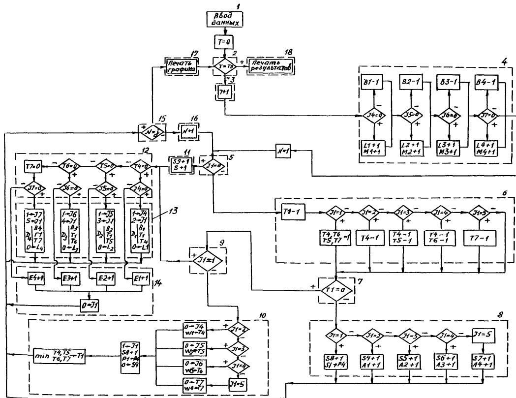
Рис.20. Алгоритм оперативного планирования работы экскаваторов
