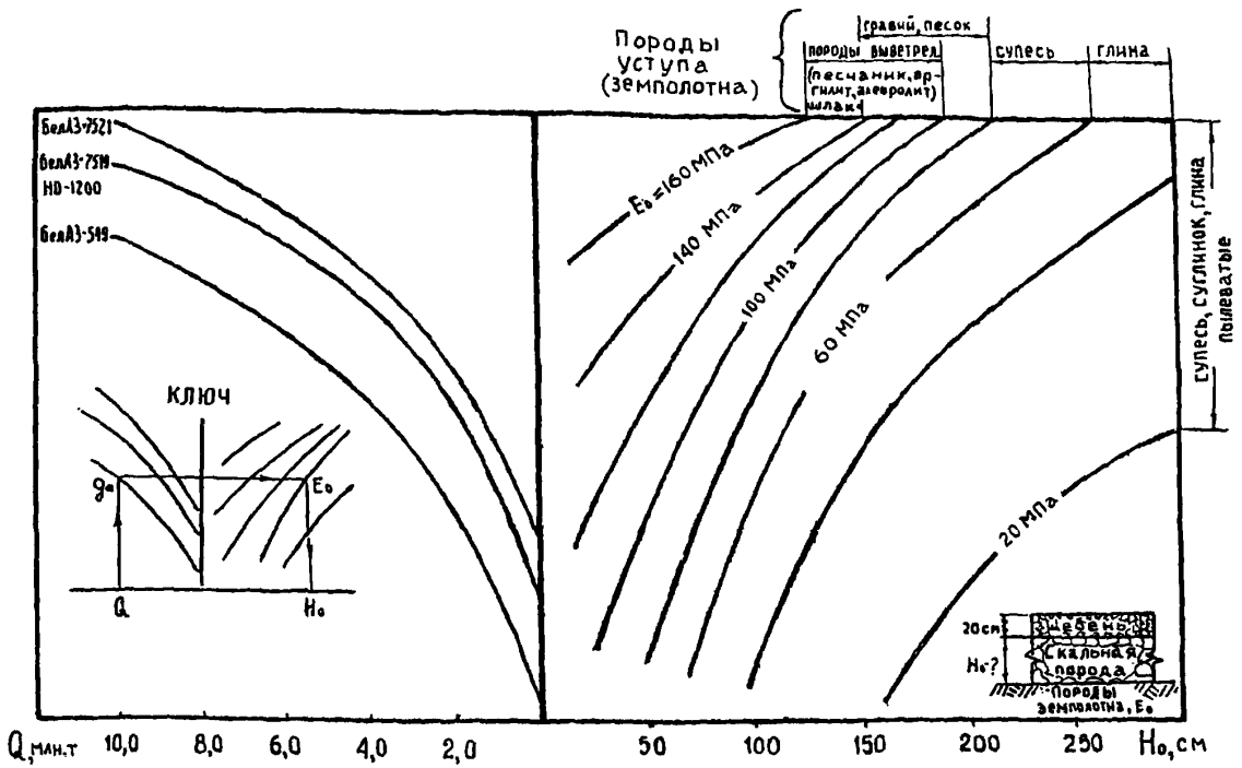
Рис. 9. Номограмма для определения толщины слоя усиления ( H_0 ) дорожных конструкций на полускальных и рыхлых породах
