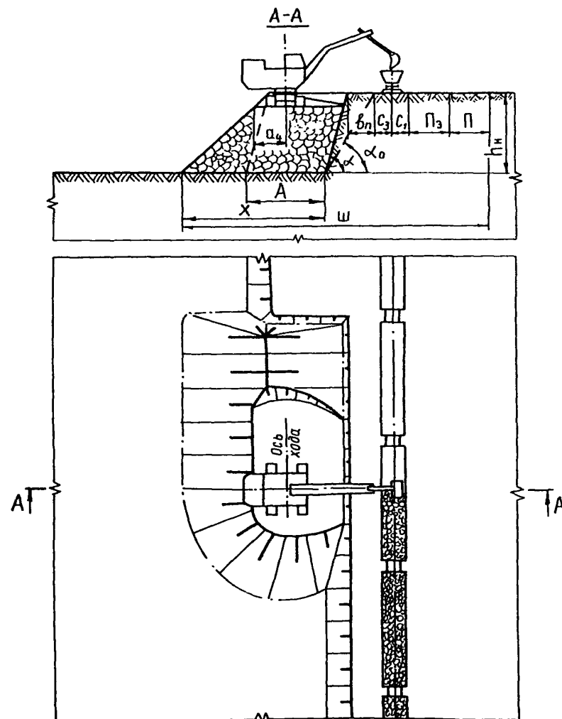
Технология разработки уступа обратной лопатой
