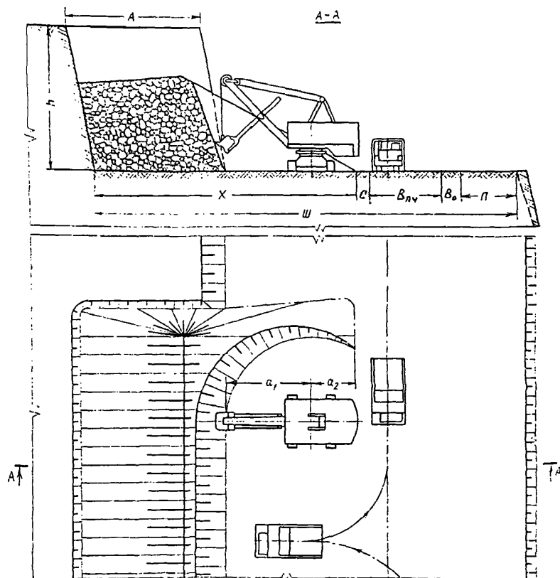
Технология разработки уступа за два прохода
