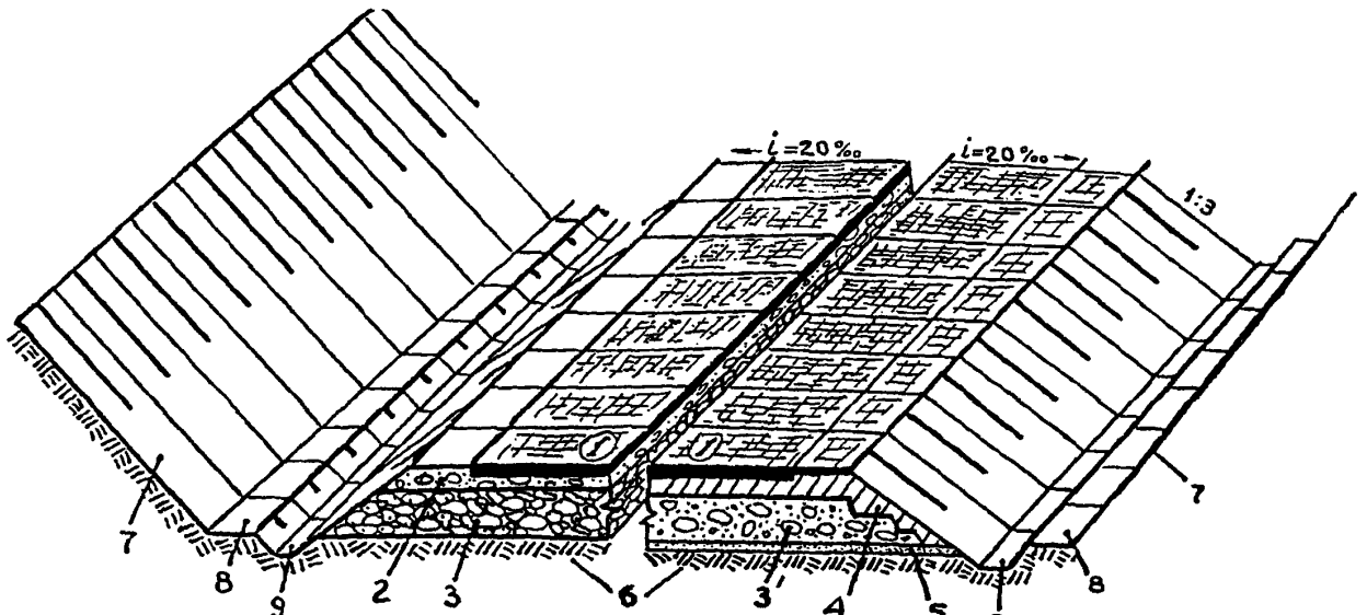
Рис. 10. Вариант дорожной конструкции, сооружаемой на горизонтах с рыхлыми породами 1 - покрытие; 2 - переходный слой; 3 - скальные породы; 3 - полускальные породы; 4 - защитный слой из глинистых грунтов; 5 - капилляропрерывающий слой; 6 - суглинок; 7 - откос уступа; 8 - закуветная полка; 9 - ковет.
