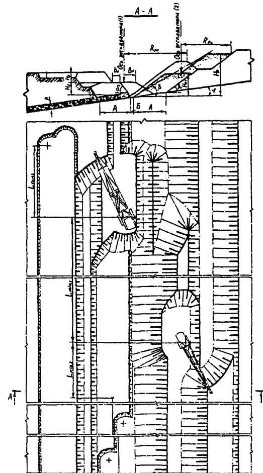
Технология разработки уступов двумя драглайнами
