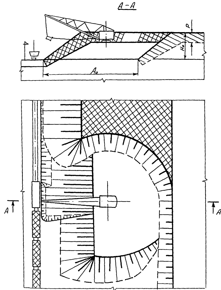
Рис. 16. Технология укладки ПШ на отвал драглайном
