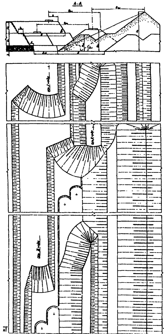
Технология разработки уступа двумя подступами широкой верхней заходкой
