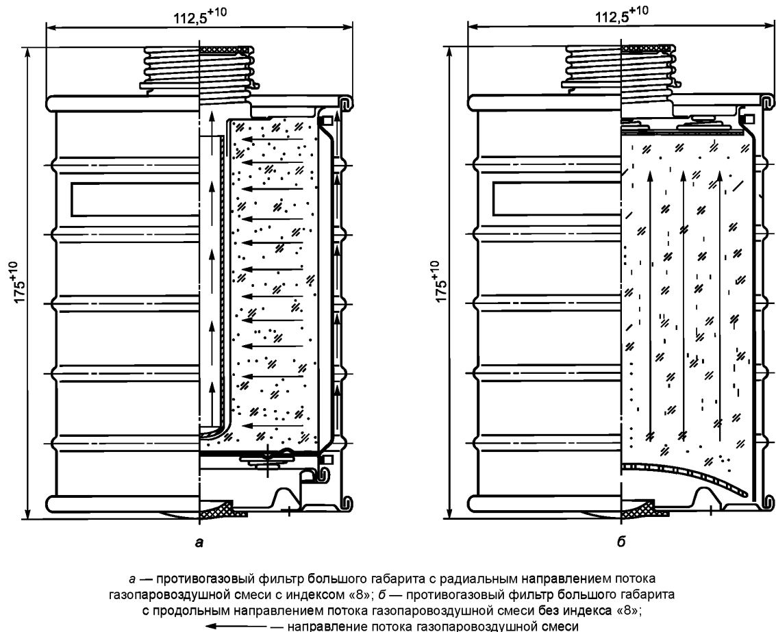
Рисунок 1 — Конструктивные исполнения противогазовых фильтров большого габарита
