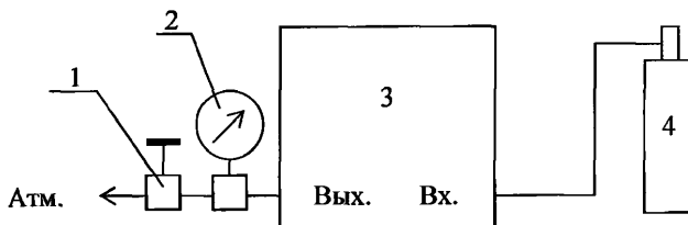
Рисунок 1. Схема поверки
