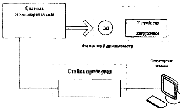
Рисунок 7 – Схема проверки ИК силы от тяги двигателя
