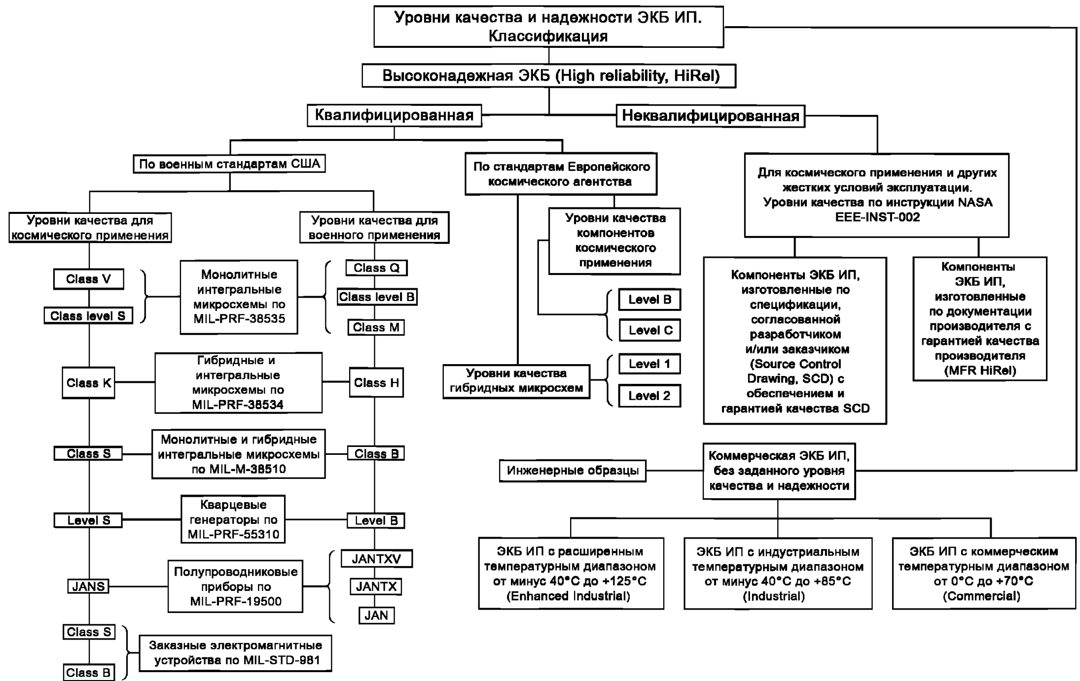
Рисунок А.1 — Уровни качества изделий (компонентов) ЭКБ ИП
