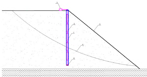
1-датчики, объединённые в цепь; 2-инклинометрическая труба; 3- блок сбора и передачи данных; 4- поверхность обрушения; 5 -откос; 6-анкер
