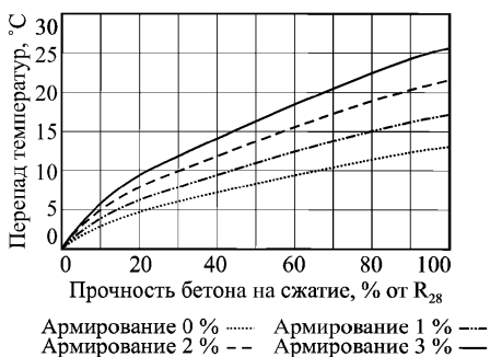
Рисунок 17.1 – Допустимый перепад температуры по сечению бетона
