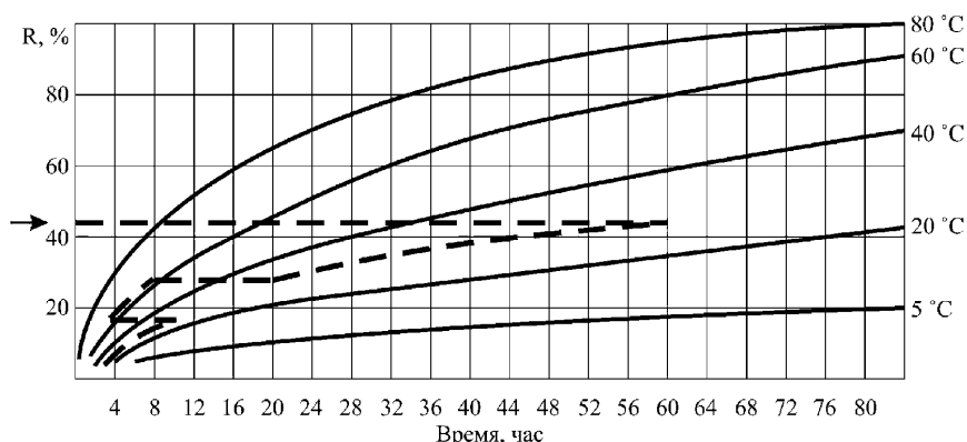
Рисунок К.2. Температурный график
