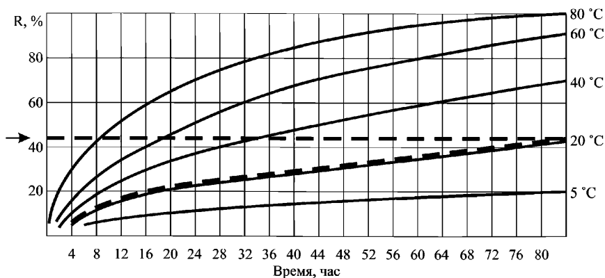
Рисунок К.3. Температурный график
