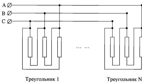
Рисунок 7.2 – Схема соединения проводов треугольником
