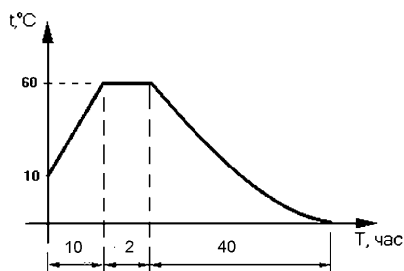
Рисунок К.1 – Температурный режим твердения бетона
