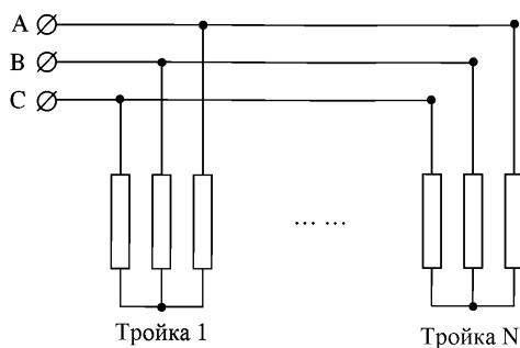
Рисунок 7.1 – Схема соединения проводов звездой
