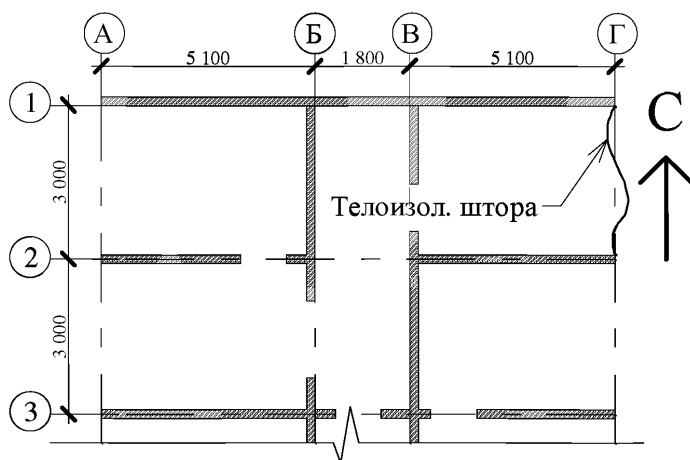
Рисунок Е.1 – Схема расположения монолитных конструкций
