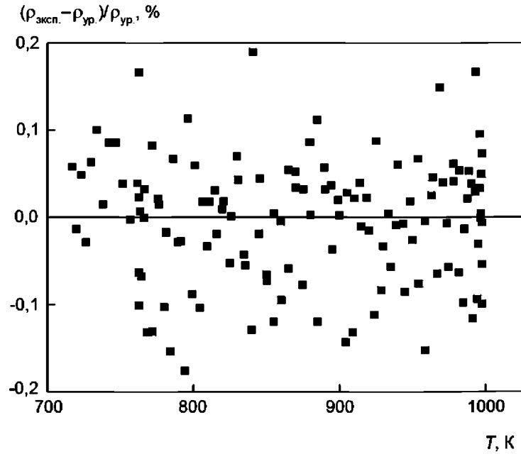
Рисунок 2 — Отклонение опытных данных настоящей работы о плотности жидкого сплава литий-свинец с содержанием 60,23 ат. % Pb от значений, рассчитанных по уравнению (1)
