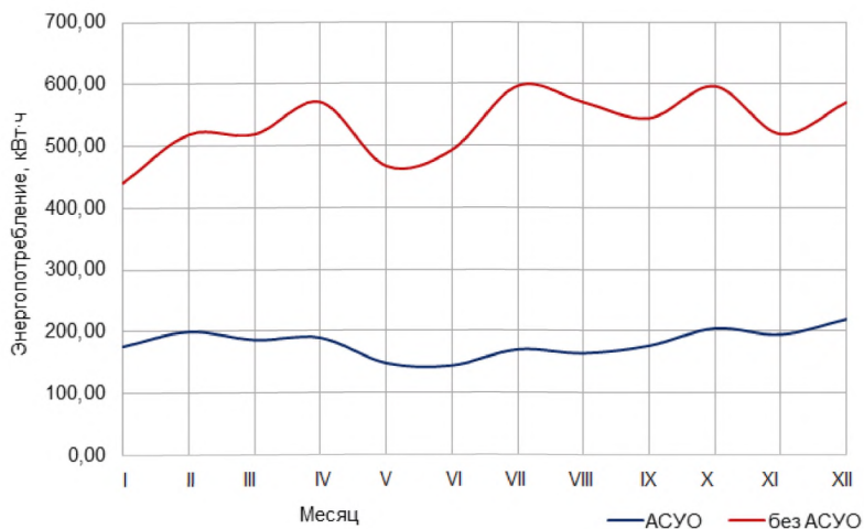
Рисунок 6.12 – Энергопотребление ОУ в месяц
