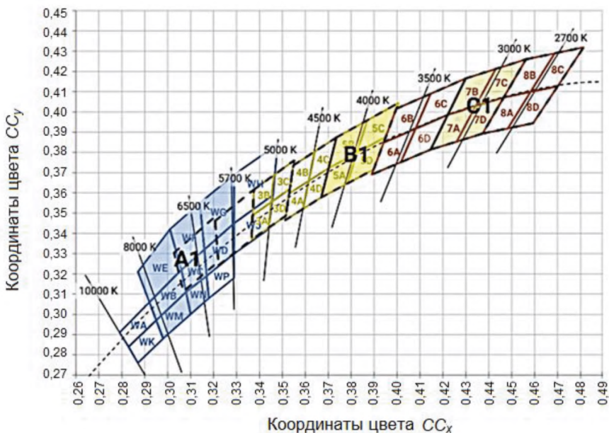
Рисунок 4.14 – Области цветности
