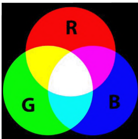
Рисунок 4.18 – Аддитивное смешивание цветов
