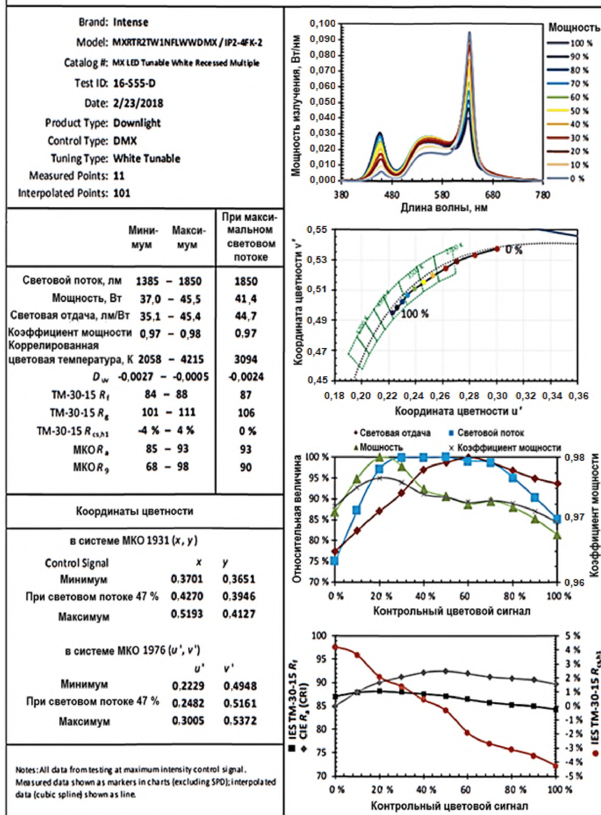
Рисунок 4.20 – Результаты тестирования светильника компании Intense Lighting
