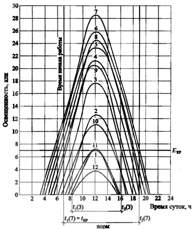
Рисунок 6.6 – Естественная освещенность в течение суток в разные месяцы года на широте Москвы
