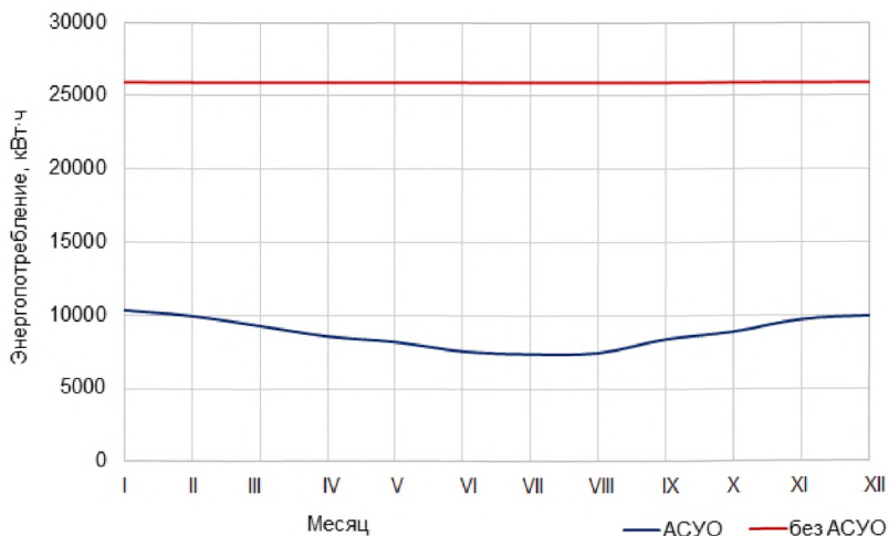
Рисунок 6.11 – Дневное энергопотребление ОУ по месяцам
