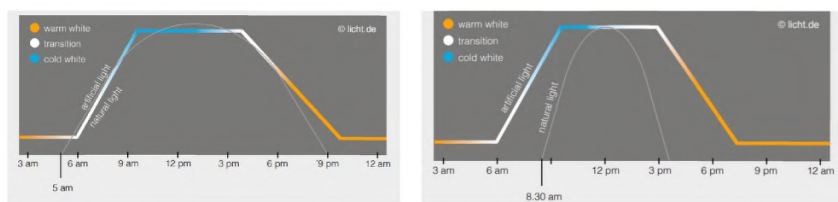
Рисунок 7.5 – Пример корреляции параметров естественного и искусственного освещения в помещении в летний и зимний периоды
