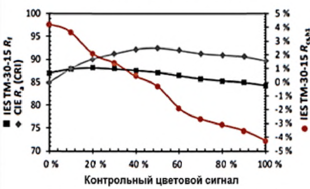
Рисунок 4.20 – Результаты тестирования светильника компании Intense Lighting
