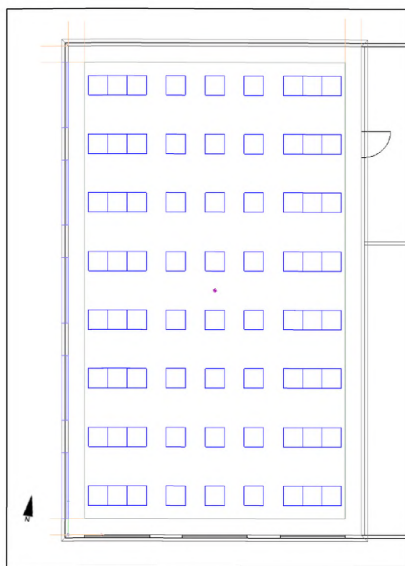
Рисунок 6.10 – Расположение ОП в помещении
