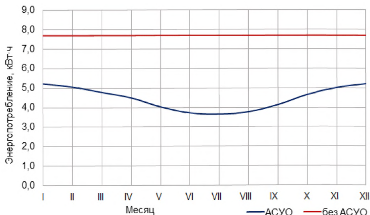
Рисунок 6.7 – Дневное энергопотребление
