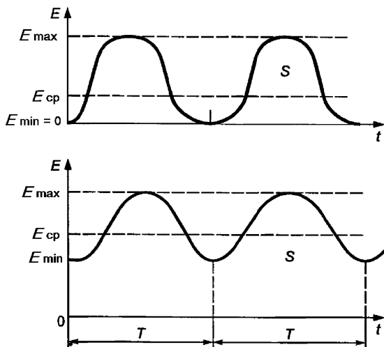
Рисунок 4.3 – Определение коэффициента пульсации освещенности
