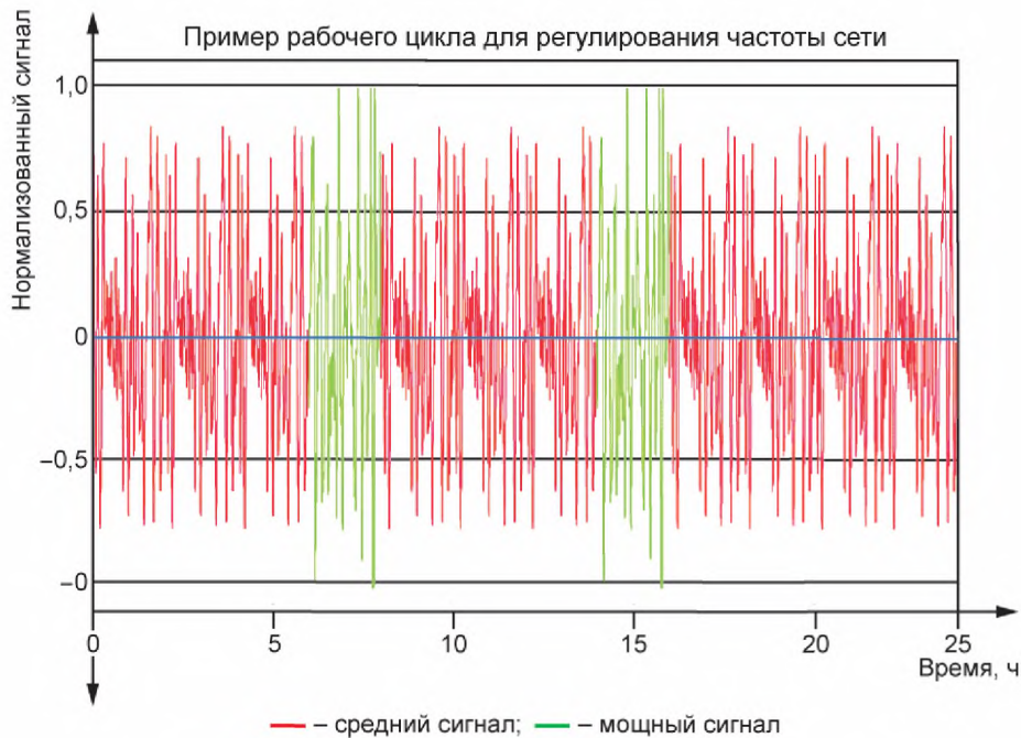
Рисунок А.1 — Рабочий цикл для приложений СНЭЭ класса А
