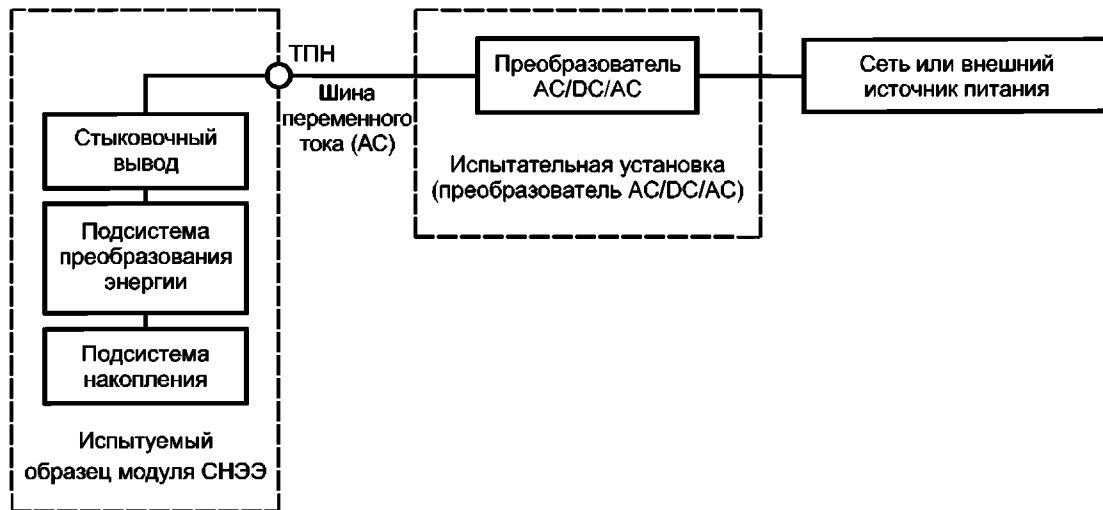
Рисунок С.2 — Схема проведения испытания методом взаимной нагрузки (с преобразователем AC/DC/AC в качестве испытательной установки)
