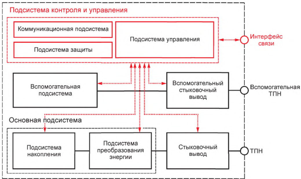
Рисунок 3 — Типовая архитектура СНЭЭ со вспомогательной ТПН
