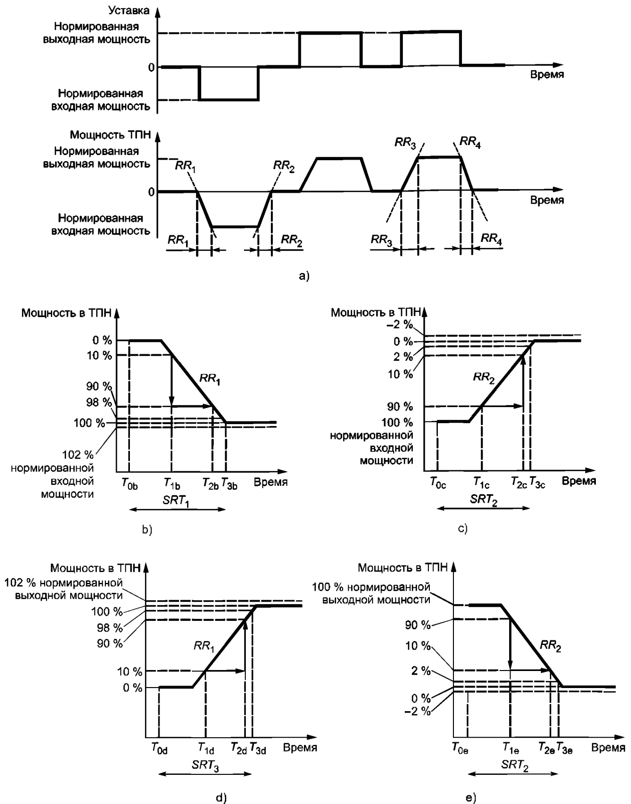
Рисунок 7 — Испытание для определения отклика системы
