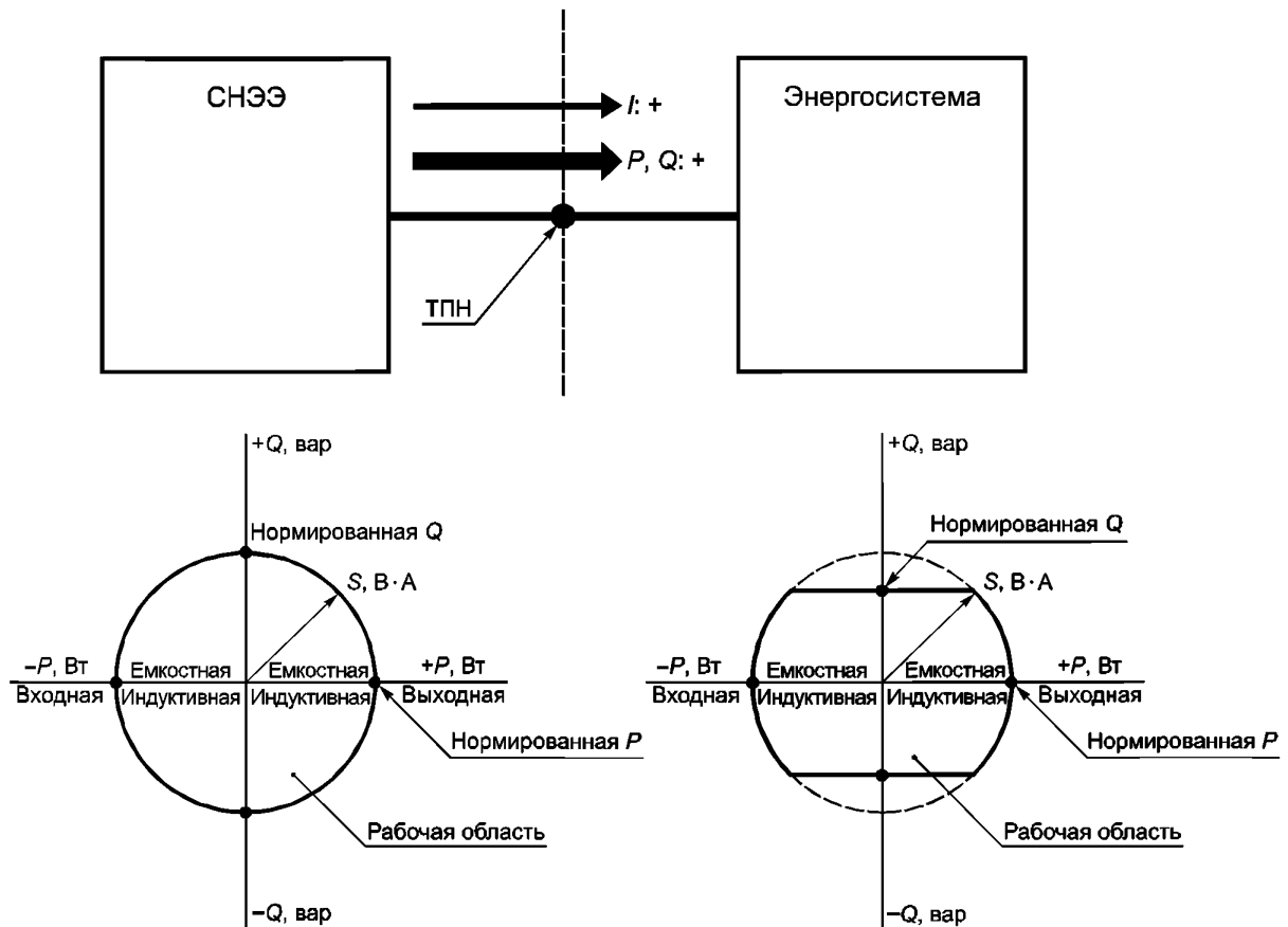
Рисунок 4 — Правило определения направления потоков активной и реактивной мощностей
