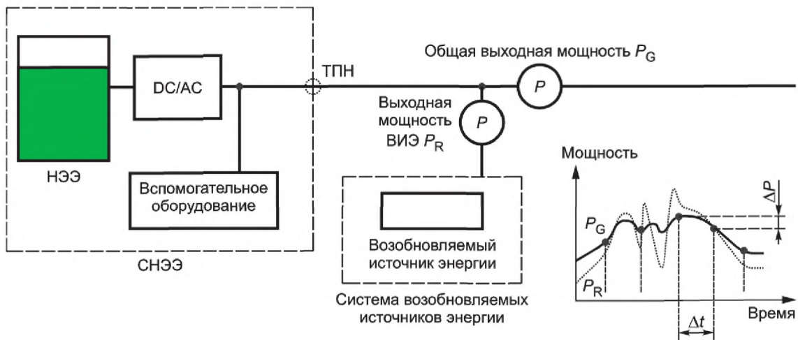
Рисунок В.1 — Испытание на компенсацию колебаний мощности
