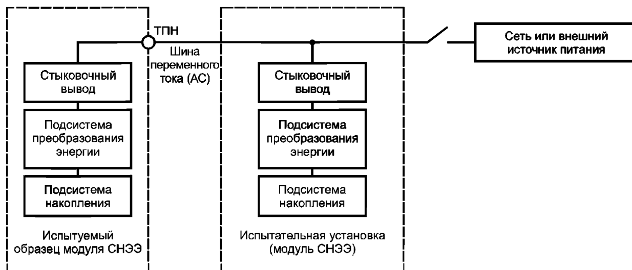
Рисунок С.1 — Схема проведения испытания методом взаимной нагрузки (с модулем СНЭЭ в качестве испытательной установки)
