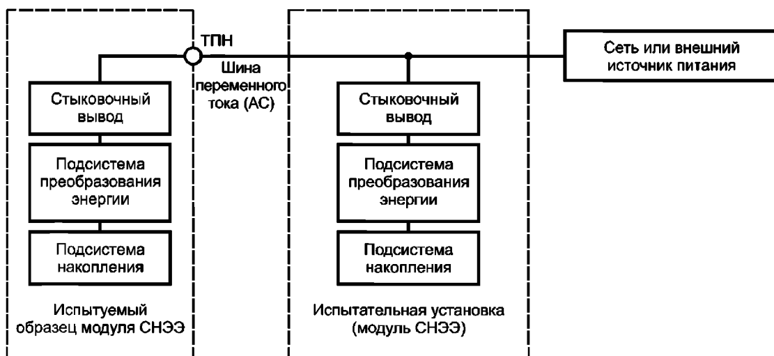
Рисунок С.3 — Схема проведения испытания методом взаимной нагрузки (с модулем СНЭЭ в качестве испытательной установки)
