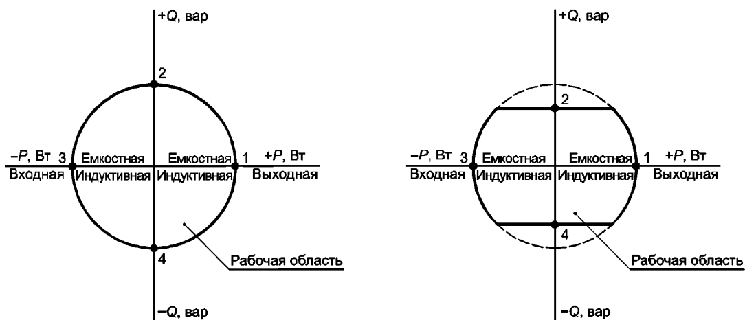
Рисунок 6 — Типовые контрольные точки для испытания при полной мощности
