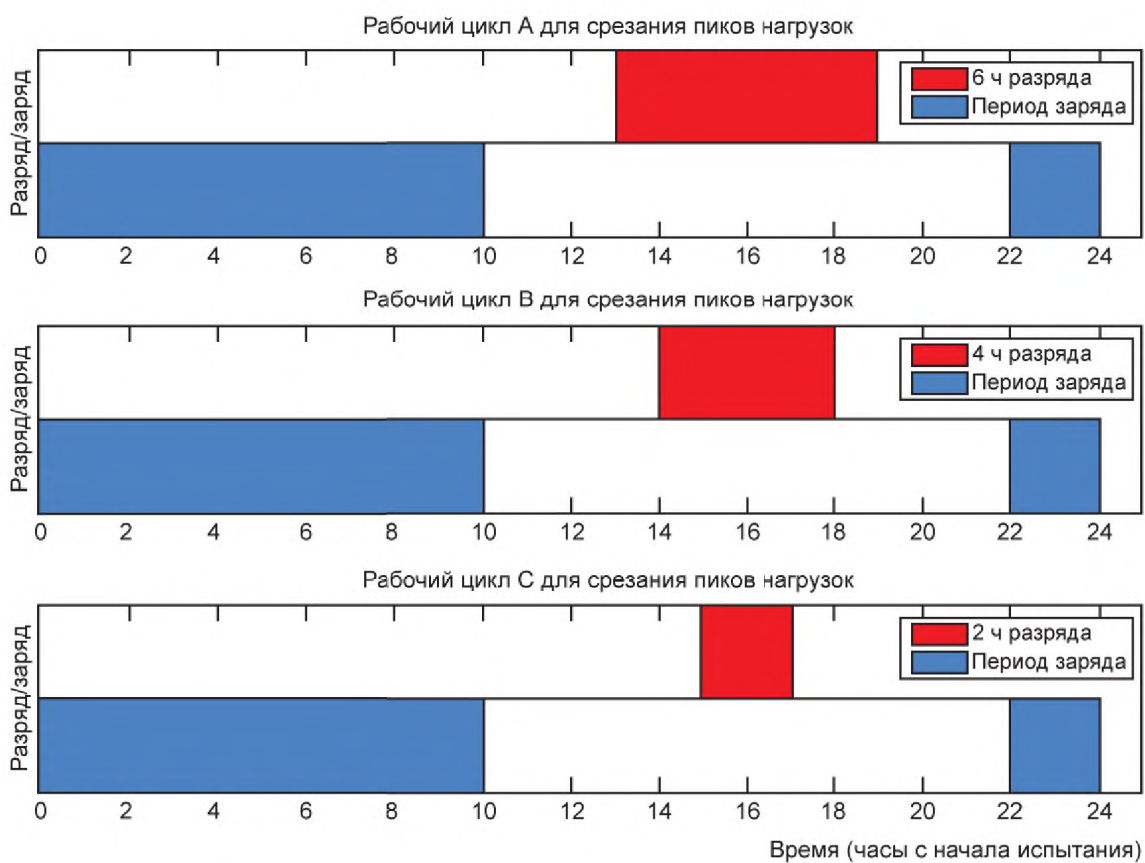
Рисунок А.2 — Рабочие циклы для приложений СНЭЭ класса В
