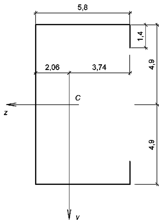
Рисунок А.3 — Расчетная схема сечения, см
