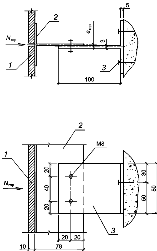
1 — облицовка; 2 — направляющая; 3 — кронштейн
