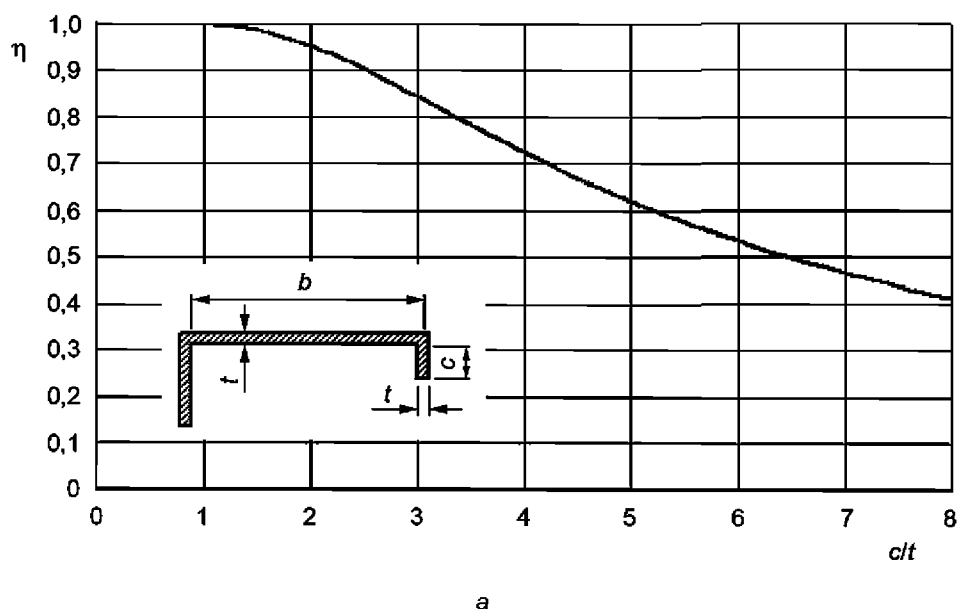
Рисунок 6, лист 1 — Значения \eta для подкрепленных элементов сечений
