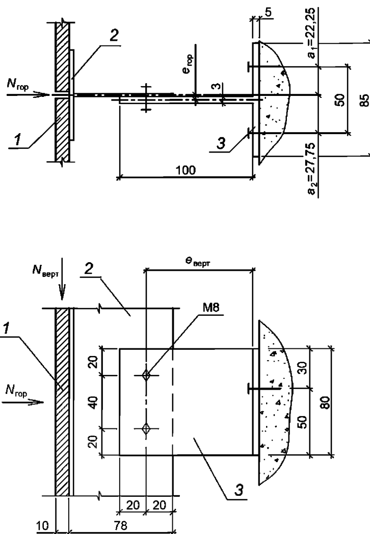
1 — облицовка; 2 — направляющая; 3 — кронштейн
