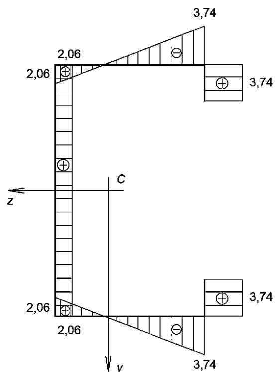
Рисунок А.4 — Эпюра координат z , см
