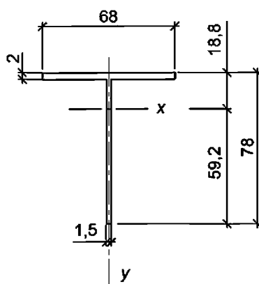
Рисунок Б.1 — Расчетное сечение направляющей
