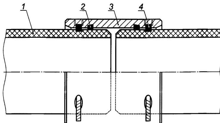
1 — труба; 2 — уплотнительное эластомерное кольцо; 3 — муфта; 4 — прут-фиксатор
