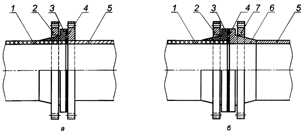
а — с фиксированным фланцем; б — со свободным фланцем; 1 — стеклокомпозитная труба; 2 — свободный стеклокомпозитный или стальной фланец; 3 — стеклокомпозитный борт; 4 — прокладка; 5 — труба из стали, чугуна или полиэтилена; 6 — полиэтиленовый борт; 7 — свободный фланец
