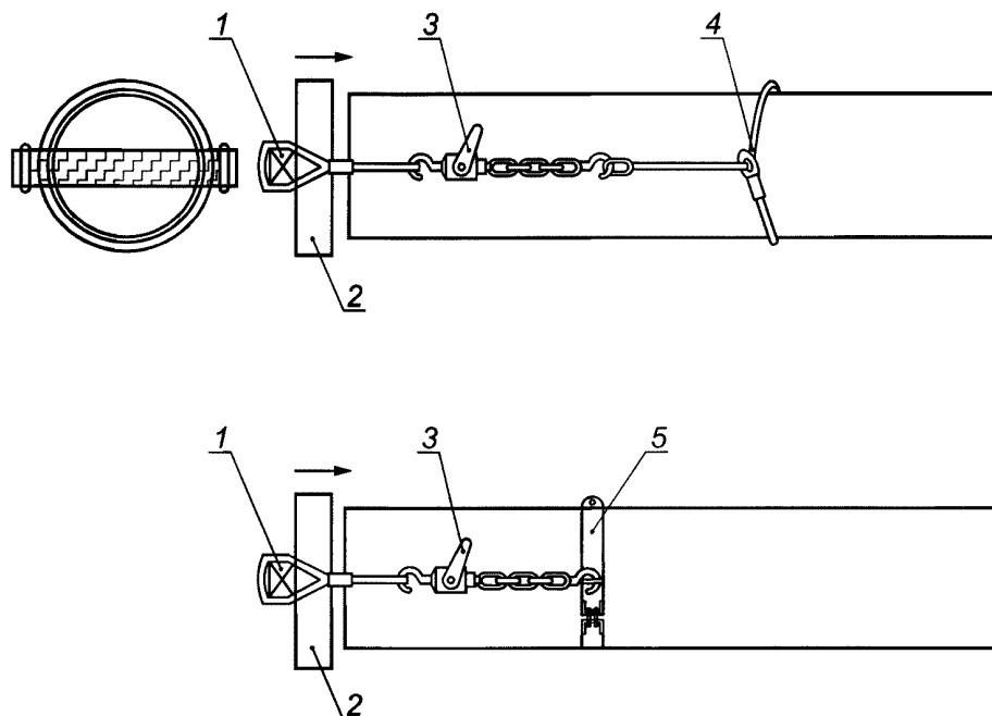
1 — брус 50 × 100; 2 — муфта; 3 — ручная (рычажная) таль; 4 — строп или канат; 5 — стальной хомут
