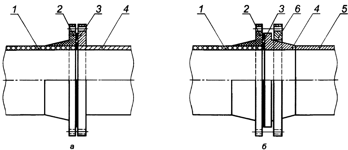
а — с фиксированным фланцем; б — со свободным фланцем; 1 — стеклокомпозитная труба; 2 — фиксированный стеклокомпозитный фланец; 3 — прокладка; 4 — труба из полиэтилена; 5 — полиэтиленовый борт; 6 — свободный фланец
