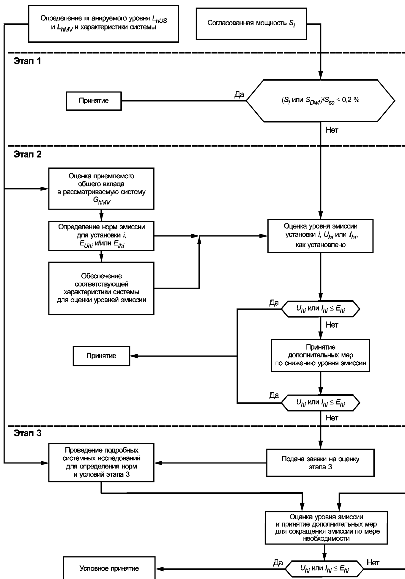
Рисунок 5 — Схема процедуры оценки при среднем напряжении
