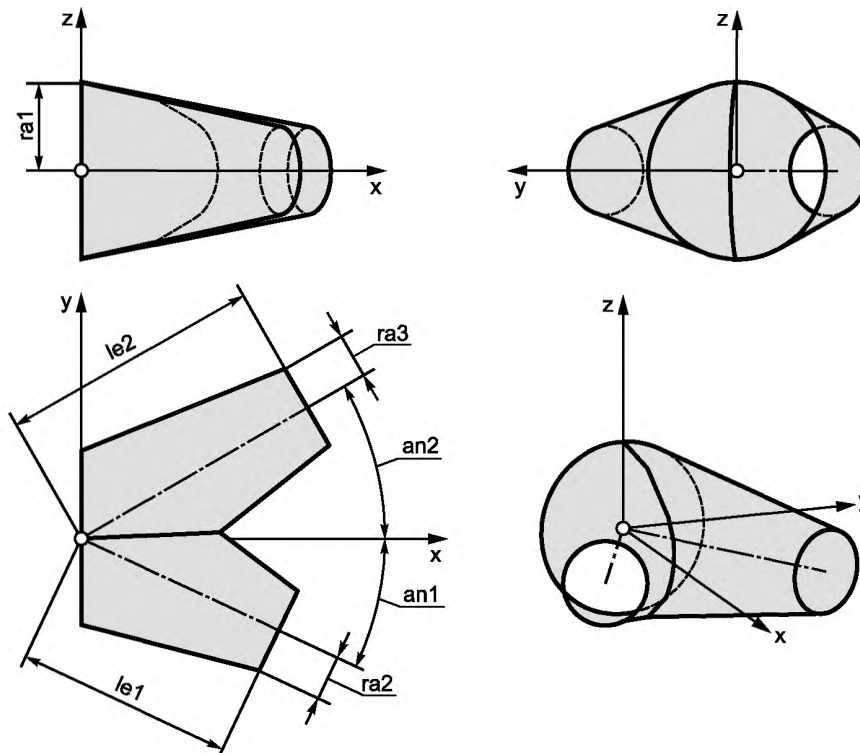
Рисунок А.20 — Y-тройник круглой трубы
