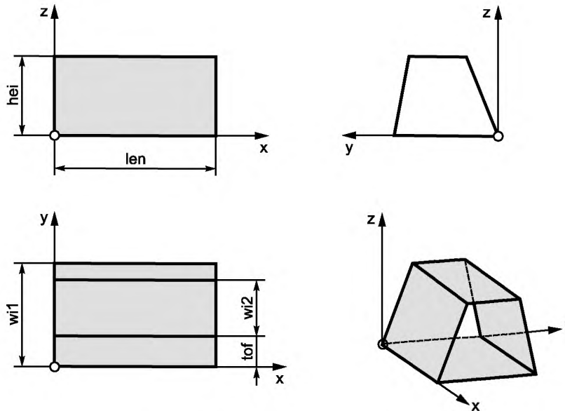
Рисунок А.10 — Трапециевидный короб
