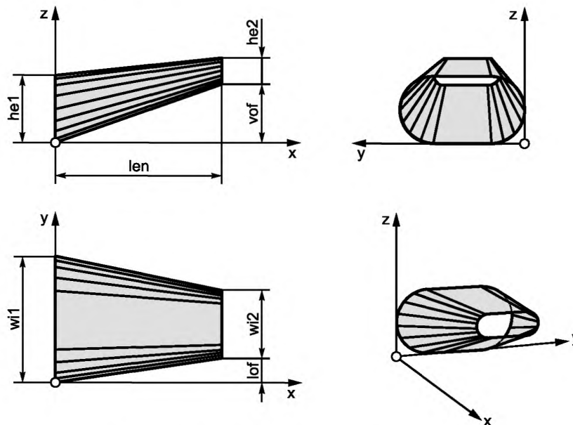
Рисунок А.13 — Переходник овального короба
