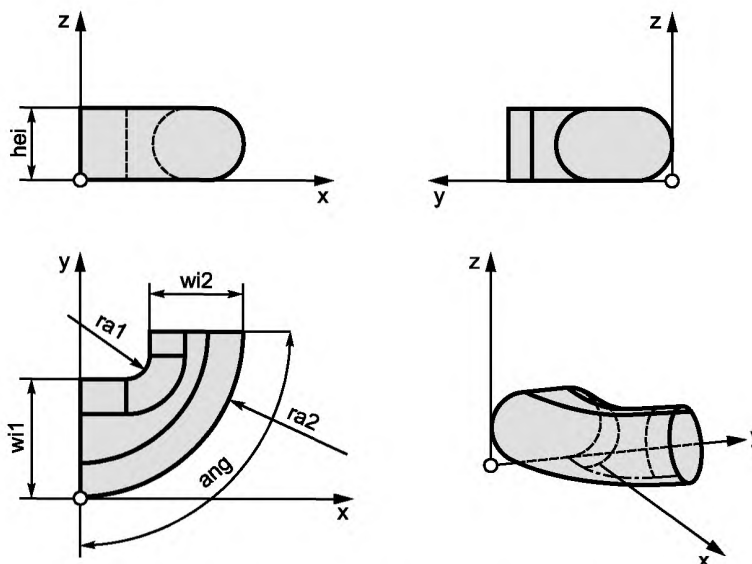
Рисунок А.14 — Изгиб овального короба
