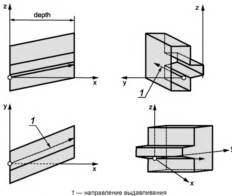
Рисунок А.21 — Выдавленная грань короба
