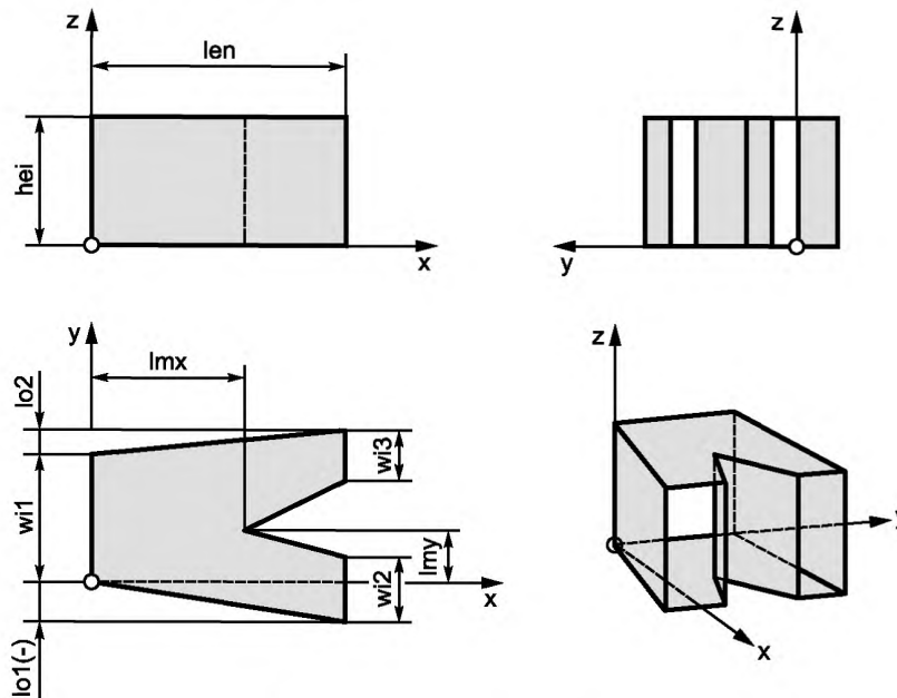
Рисунок А.7 — Y-тройник прямоугольного короба
