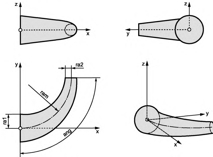
Рисунок А.2 — Тороидальный изогнутый переходник
