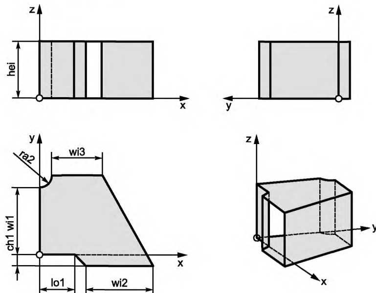
Рисунок А.6 — Тройник прямоугольного короба
