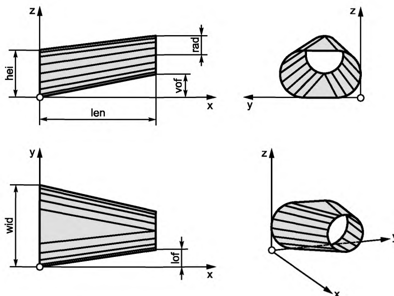
Рисунок А.15 — Овальный/круглый переходник
