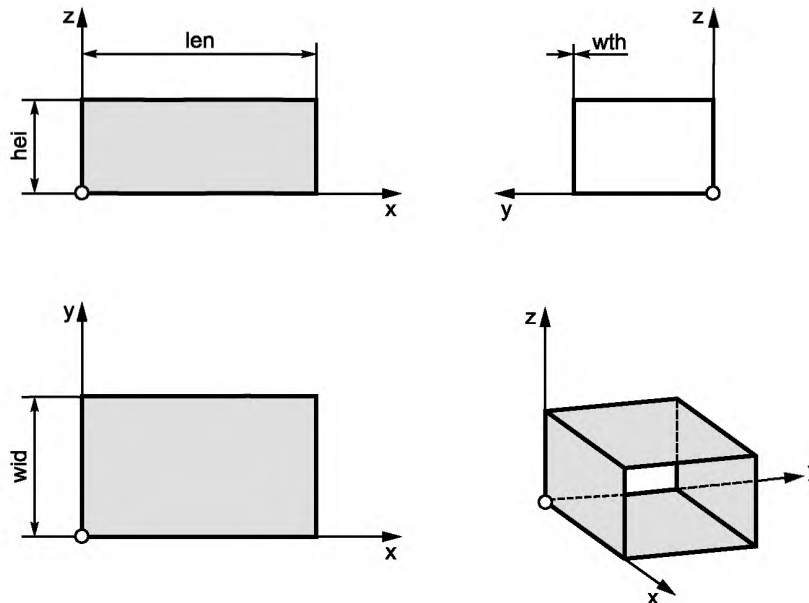
Рисунок А.3 — Прямоугольный короб
