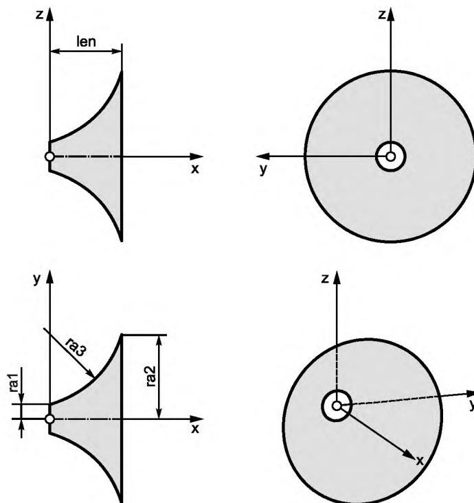
Рисунок А.18 — Радиальный переходник круглой трубы
