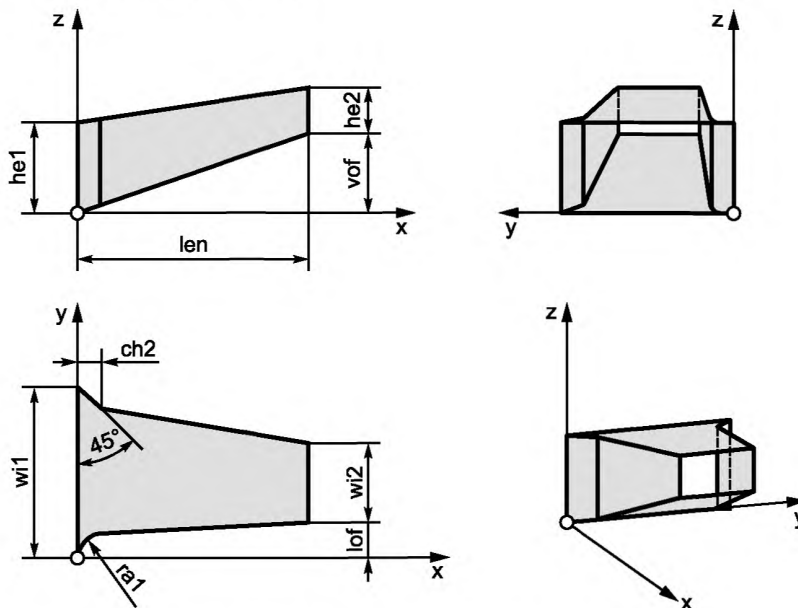
Рисунок А.4 — Переходник прямоугольного короба
