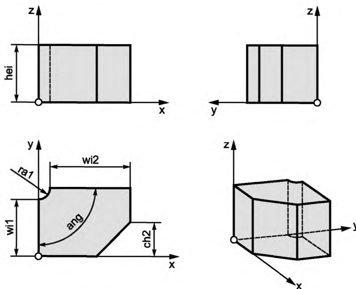
Рисунок А.5 — Изгиб прямоугольного короба
