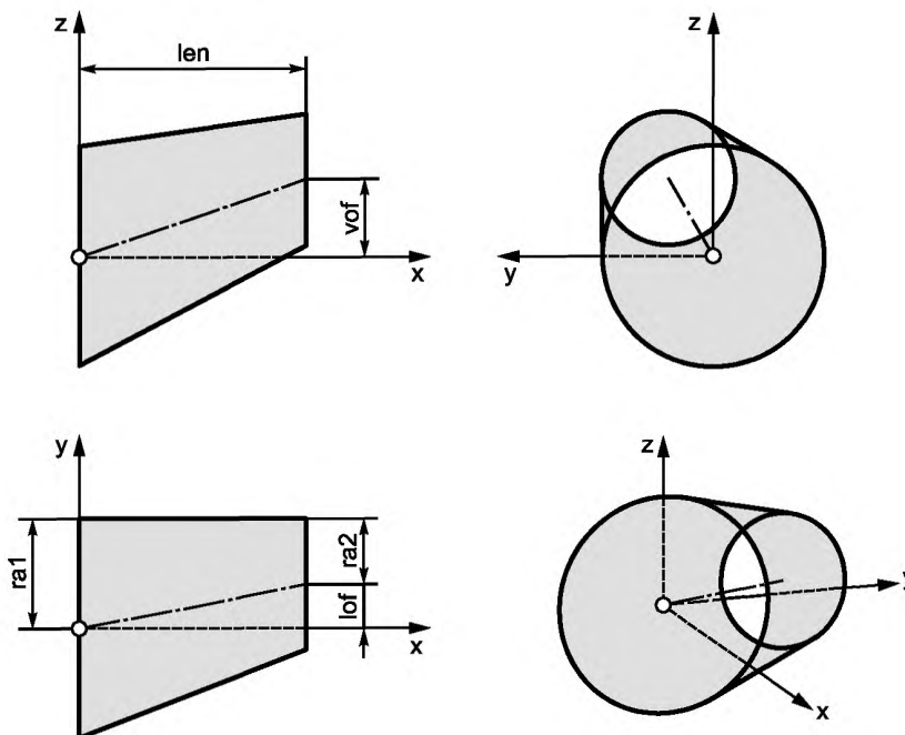
Рисунок А.17 — Переходник круглой трубы
