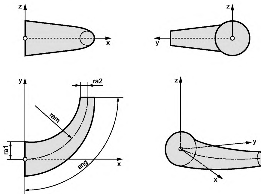
Рисунок А.19 — Изогнутый переходник круглой трубы
