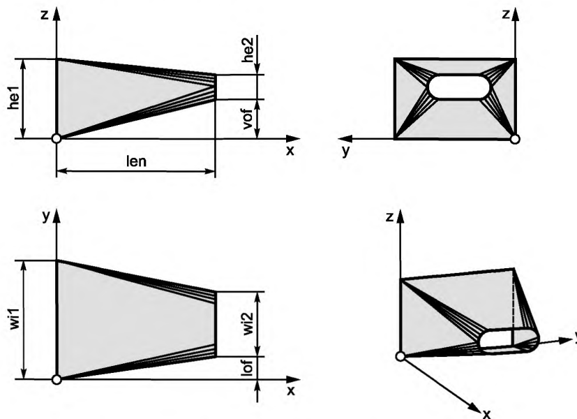
Рисунок А.8 — Прямоугольный/овальный переходник
