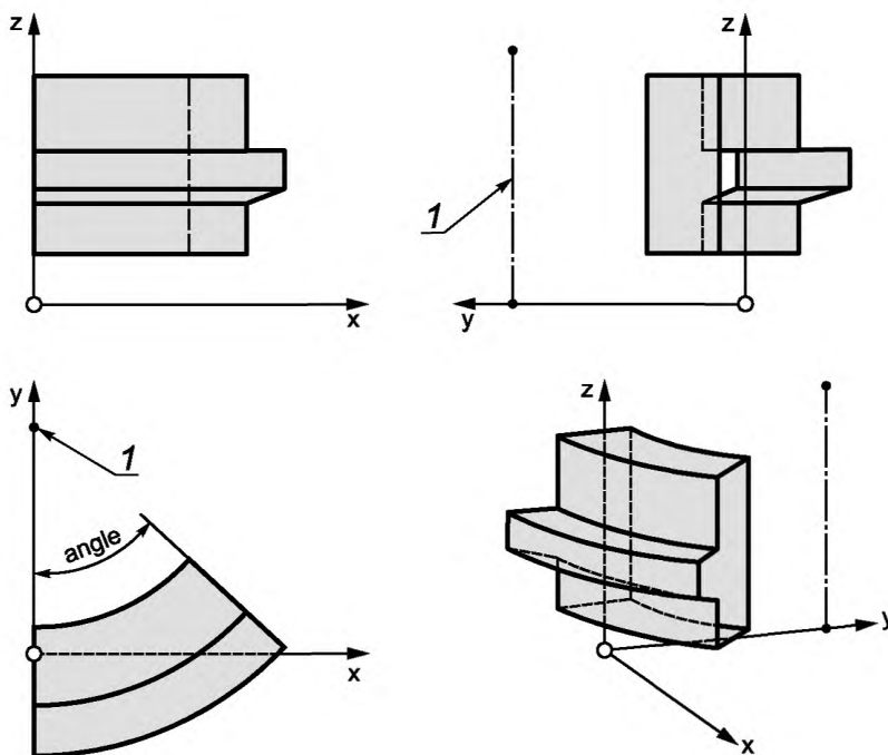
Рисунок А.22 — Вращение грани короба
