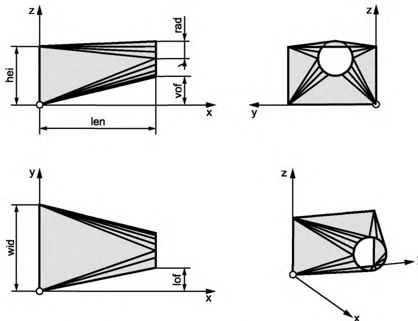
Рисунок А.9 — прямоугольный/круглый переходник
