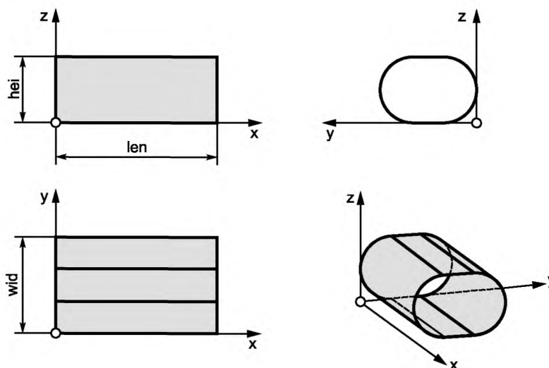
Рисунок А.12 — Овальный короб
