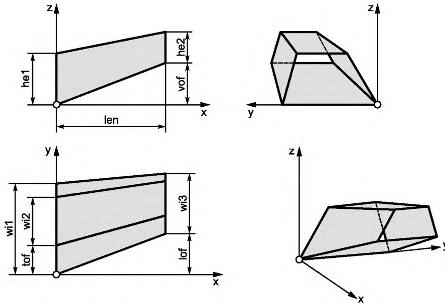
Рисунок А.11 — Переходник трапецевидного короба
