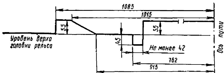
Рис. 2. Нижняя часть габарита C и C_n для двойных перекрестных стрелочных переводов
