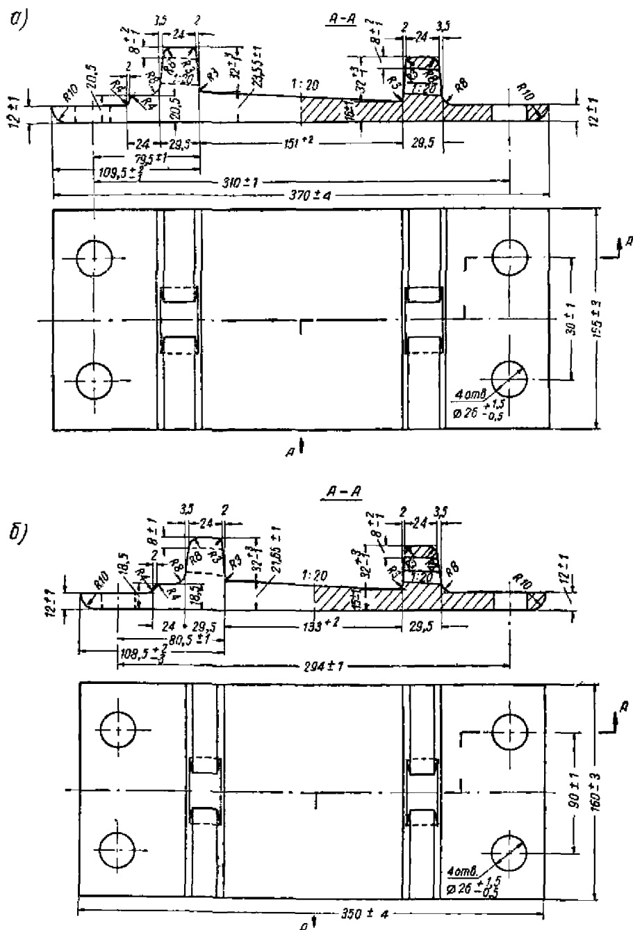
Рис. 16. Подкладки марки К клинчатые с шурупным креплением к деревянной шпале:
