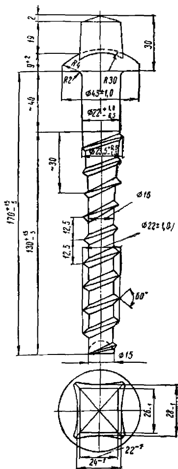
Рис. 23. Шуруп для прикрепления стрелочных переводов (вес—0,54 кг)
