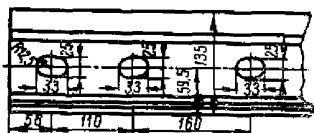
Боковой вид конца рельса
