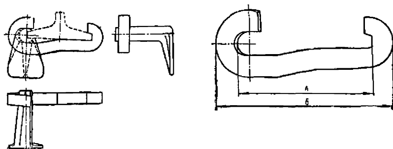
Рис. 25. Противоугонок самозаклинивающийся
