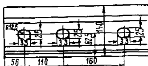
Боковой вид конца рельса
