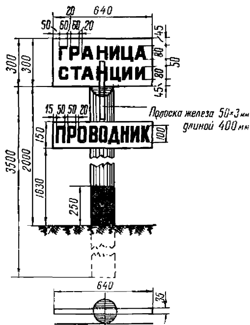
Сигнальные знаки «Граница станции» и «Проводник».
