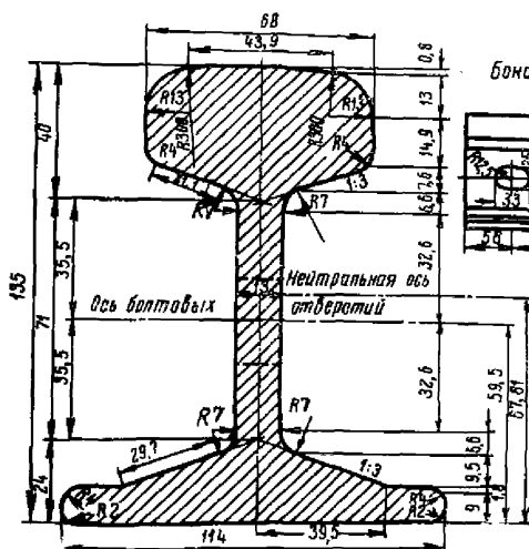
Поперечный разрез
