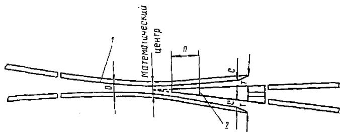
Рис. 44. Места контрольных измерений желобов крестовины:
