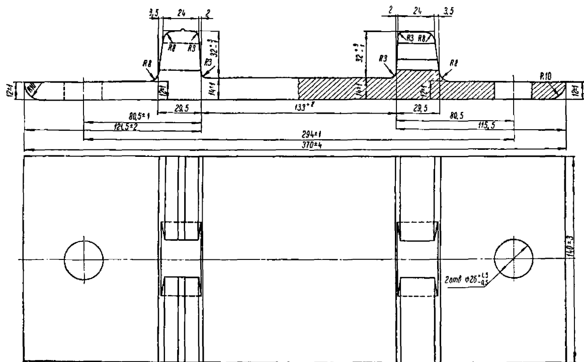
Рис. 15. Подкладка марки К плоская с шурупным креплением к железобетонной шпале и расположением отверстий для пути с рельсами типа Р50
