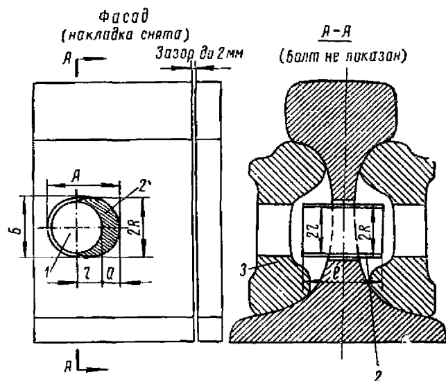
Рис. 27. Стыкование рельсов с применением вкладышей:
