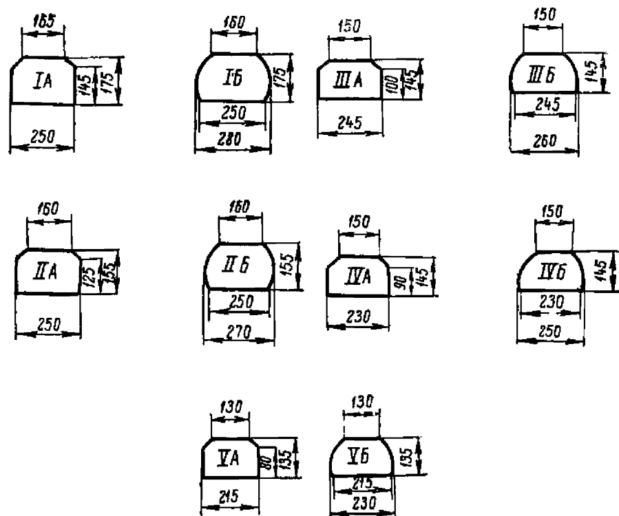
Рис. 26. Поперечные сечения шпал
