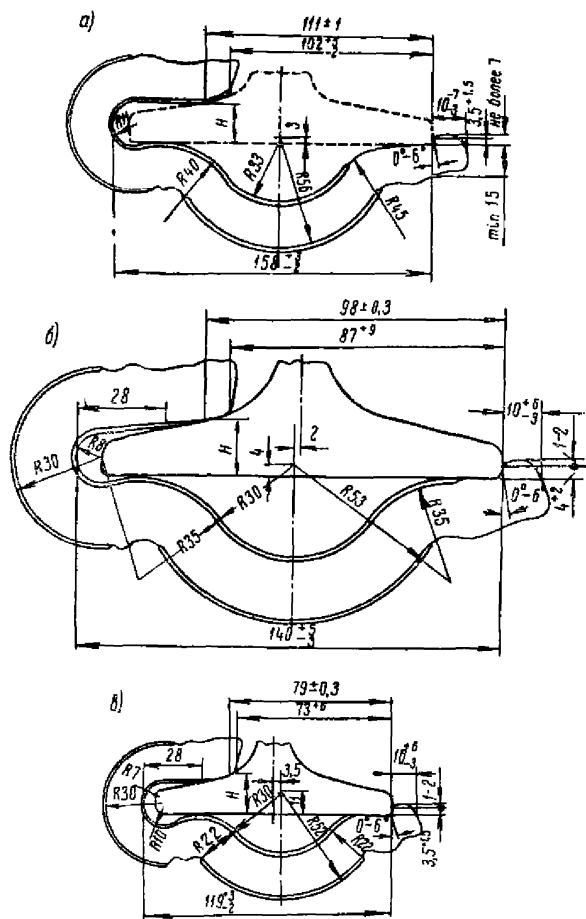
Рис. 24. Противоугоны пружинные к рельсам типа: а—Р65; б—Р50; в—Р43
