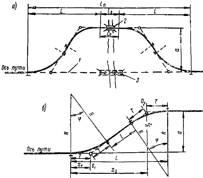
Рис. 1. Схема обхода на прямом участке основного пути: а—общая схема обхода; б—разбивка обхода: 1—постоянная трасса; 2—временный мост; 3—строющийся мост
