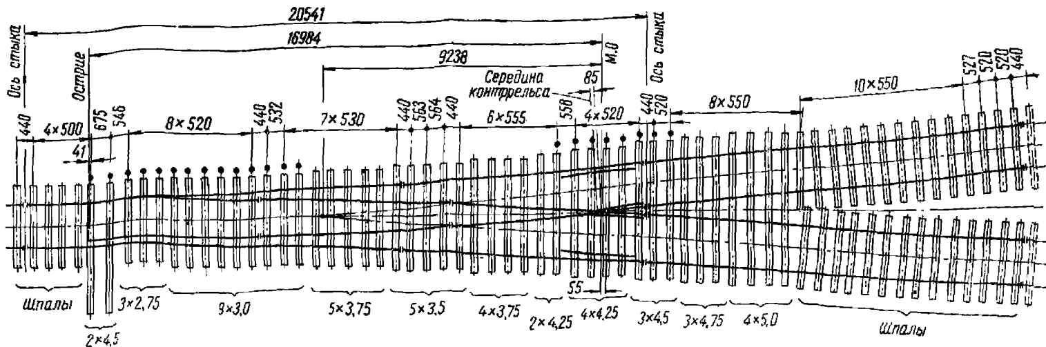
Схема разбивки
