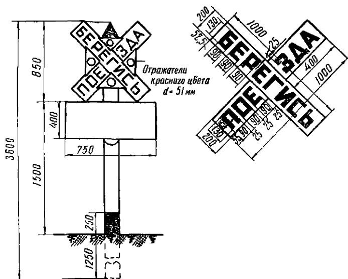
Знак «Берегись поезда» для автогужевого транспорта на неохраняемых переездах
