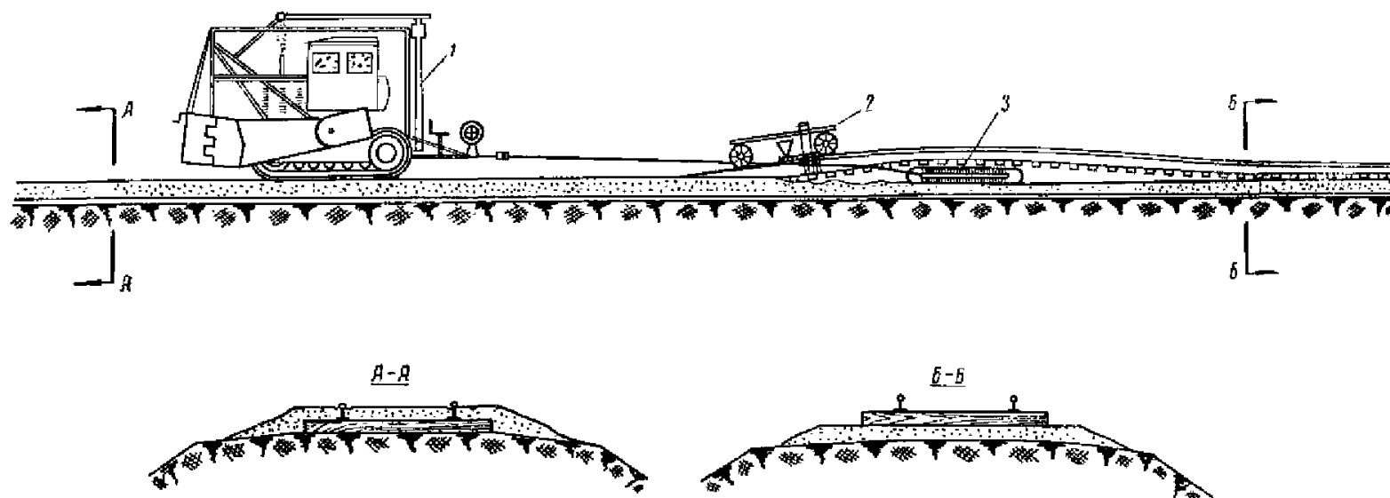
Рис. 67. Схема подъёмки пути ползучим путепо́дъёмником: 1—трактор с навесным оборудованием для дозирования балласта в путь; 2—тележка со щётками для сметания балласта со шпал; 3—ползучий путепо́дъёмник
