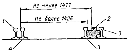
Рис. 45. Ограничение размеров на крестовине:
