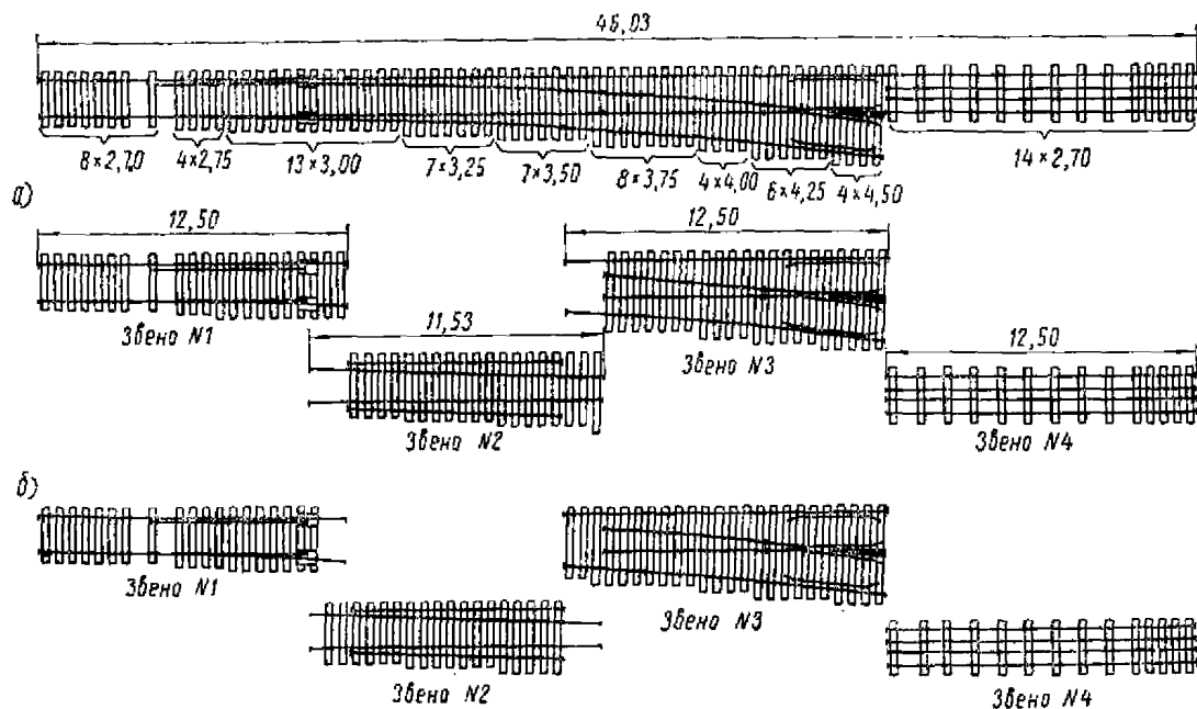
Рис. 60. Схема пришивки переводных брусьев и шпал на звеньях стрелочных переводов типов Р50 и Р43 с крестовиной марки \frac{1}{11} :
