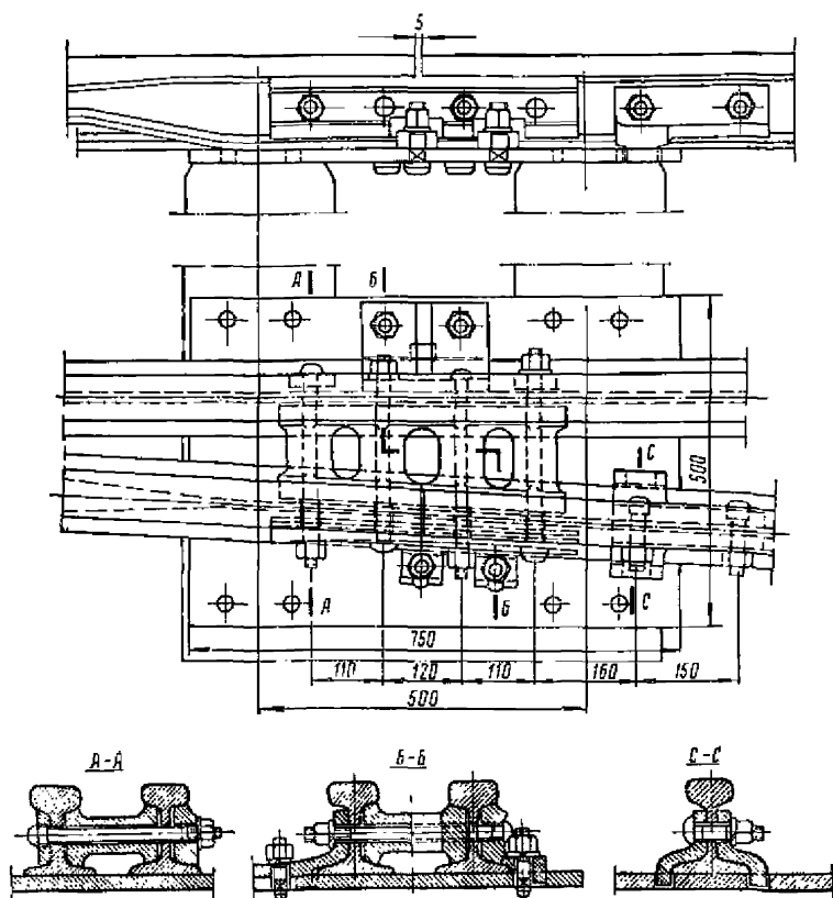
Рис. 41. Накладочное корневое крепление с выпрессовкой острижков в корне
