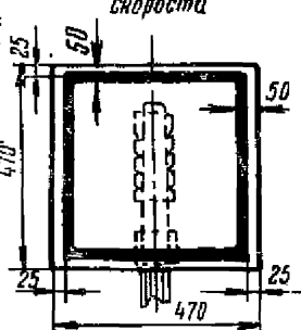
Сигнал уменьшения скорости
