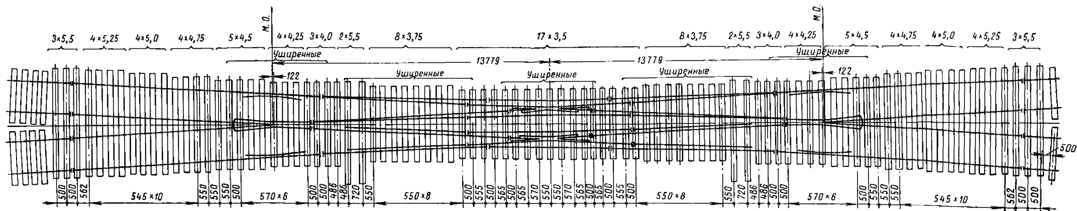
12. Эпюра двойного перекрестного стрелочного перехода из рельсов Р43 с крестовинами марки 1/9
