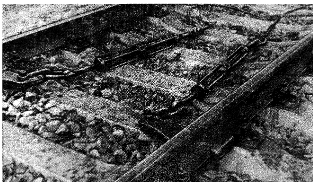
Рис. 70. Винтовые стягивающие приспособления Белорусской ж. д.
