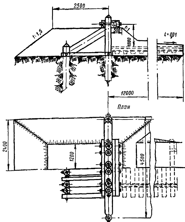
Типовая балластная призма к путевому упору
