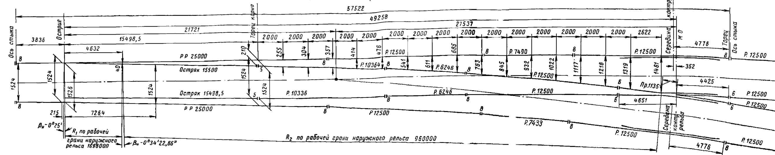
С х е м а р а з б и в к и
