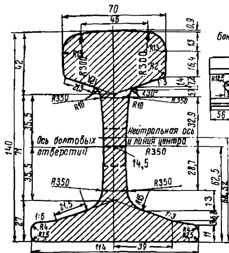
Поперечный разрез
