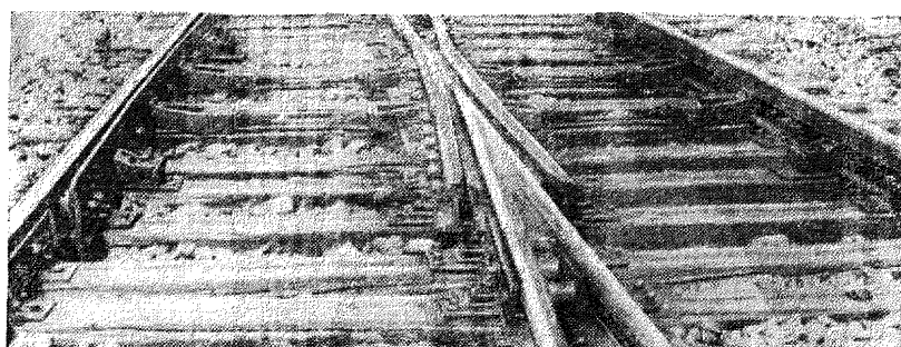
Рис. 42. Крестовина с сердечником типа общей отливки с изнашиваемой частью усовиков, высокими контрельсами и распорками
