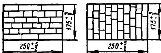
Рис. 30. Конструкция и размеры поперечных сечений клееных переводных брусев
