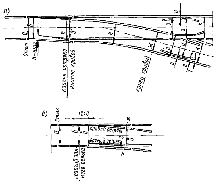
Рис. 43. Места измерений ширины колеи в стрелочных переводах: а—с прямыми острьяками; б—с кривыми острьяками
