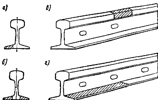
Рис. 6. Дополнительная маркировка рельсов: — а—длиной 12,46 м; б—длиной 12,42 и 24,92 м; в—с закален- ными концами; г—твёрдых рельсов
