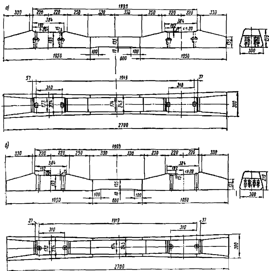
Рис. 27. Шпала струнобетонная цельнобрусковая: а—с болтовым прикреплением подкладок; б—с шурупным прикреплением подкладок
