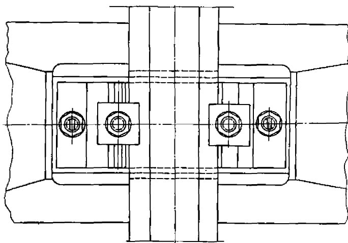
Рис. 28. Болтовое прикреплeние плоской подкладки к железобетонной шпале с изоляцией на болтах
