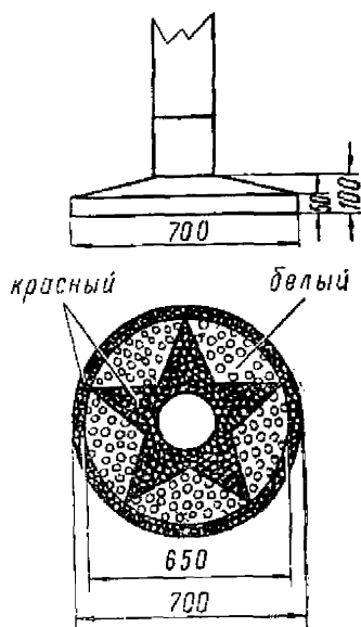
Розетка для отделки путевых знаков
