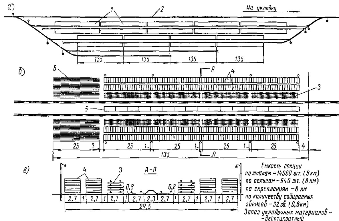
Рис. 51. Схема звеносборочной базы с применением для выгрузки материалов стреловых кранов на железнодорожном ходу:
