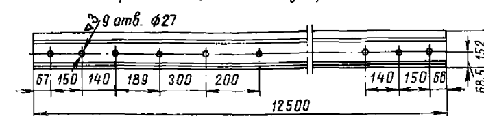
С х е м а сверления отверстий в рельсах, примыкающих к хвосту крестовины
