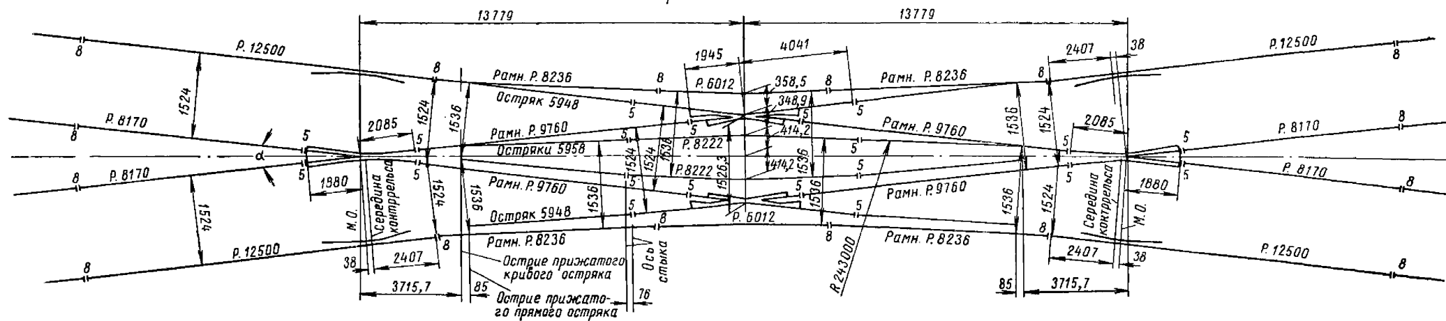
Схема разбивки
