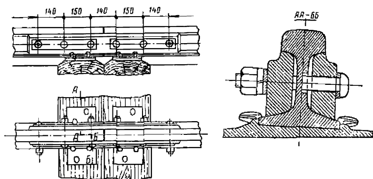
Рис. 6. Изолирующий стык рельсов типа Р50 с лигнофенолевыми накладками
