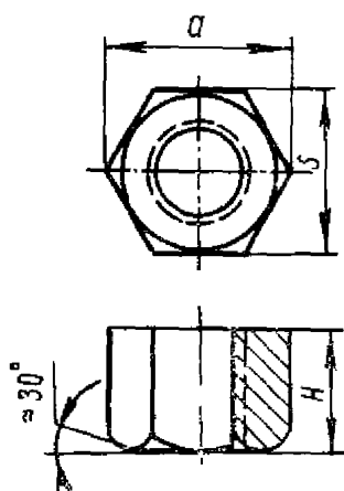
Рис. 11. Гайка
