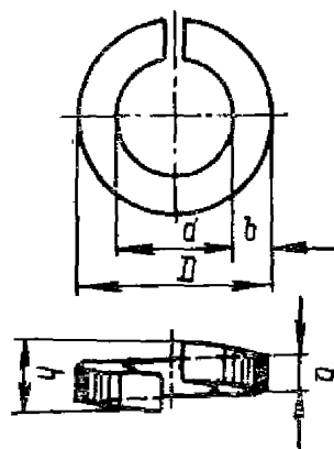
Рис. 12. Пружинная шайба
