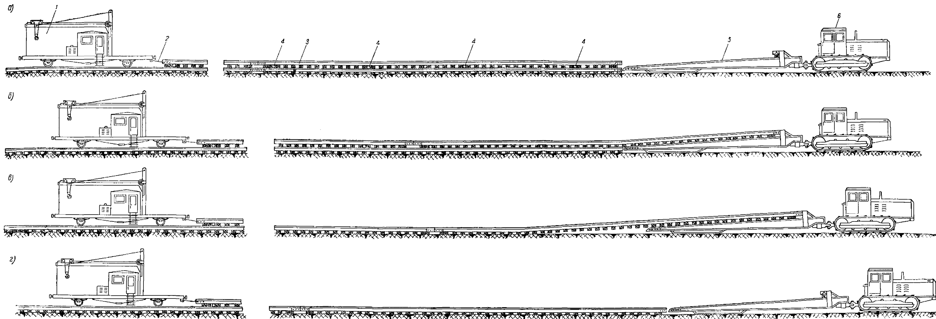
Рис. 58. Последовательность работ при укладке пути путеукладчиком ЗКУ: а—исходное положение перед укладкой; б—звено надвинуто автодрезиной на укладочную раму; в—звено пути стаскивается трактором на земляное полотно; г—укладочная рама вытаскана трактором из-под звена пути; 1—автодрезина АГМ У ; 2—упряжной треугольник; 3—укладываемое звено; 4—ролик; 5—укладочная рама; 6—трактор С-80 или С-100
