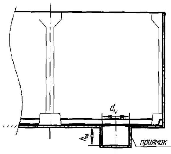
Рисунок А.5 Схема измерений параметров призмки
