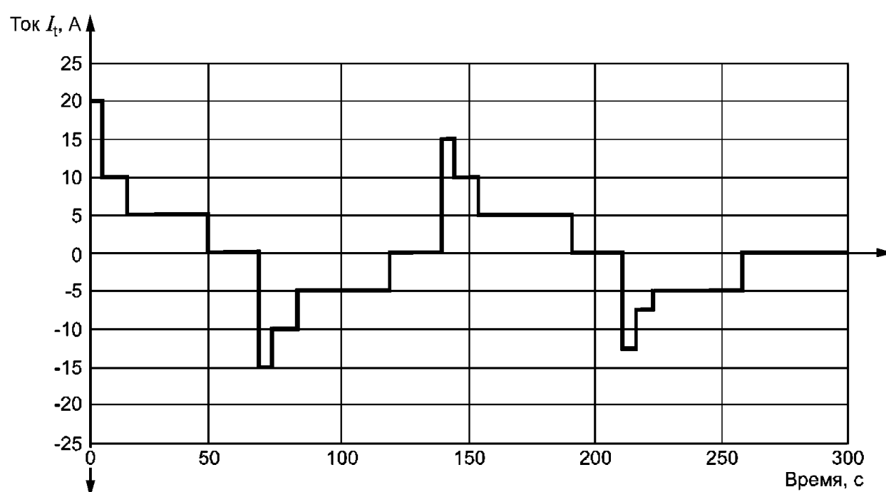
Рисунок 5 — ППР при циклировании аккумуляторов для ЭМГ
