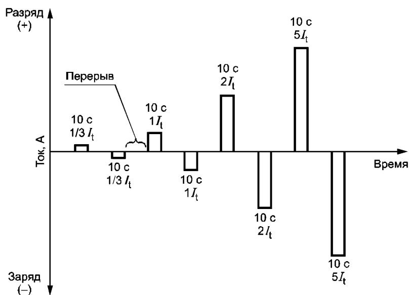
б) Порядок проведения испытания по определению ВАХ для применения ЭМА
