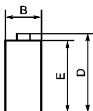
с) Призматические аккумуляторы (1)
