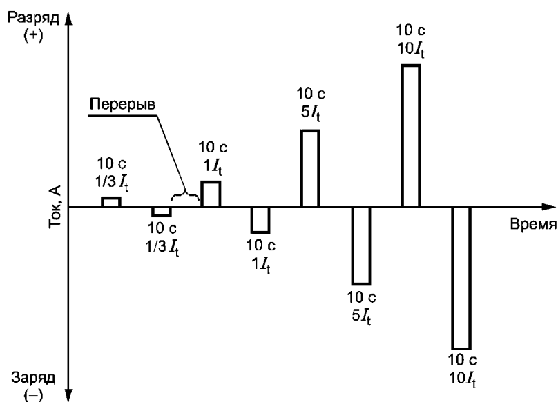
а) Порядок проведения испытания по определению ВАХ для применения ЭМГ
