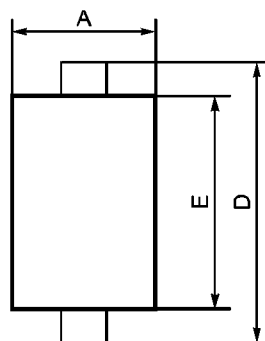
д) Призматические аккумуляторы (2)
