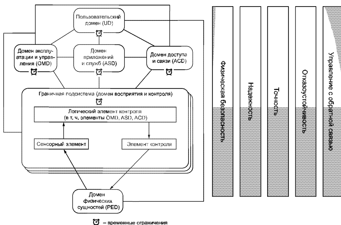
Рисунок 4 — Представление контроля системы ИВ реального времени (см. [2])
